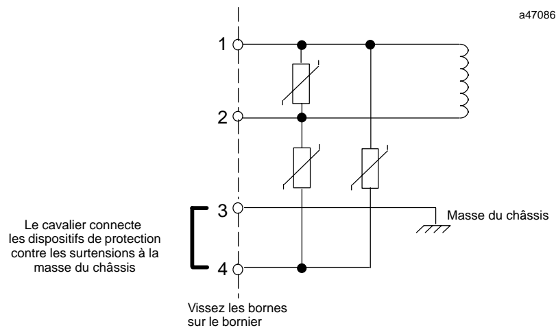
Figure 1-20. Dispositifs de protection contre les surtensions et cavalier
