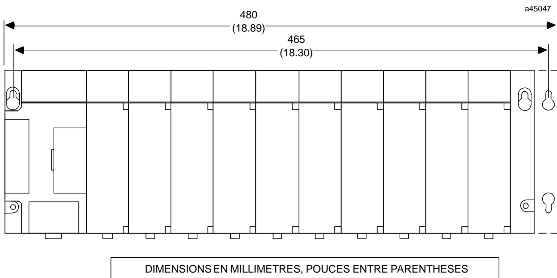
Figure 1-8. Dimensions pour le montage d'une platine dans un bac 19''
