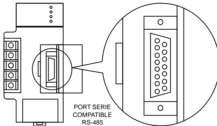
Figure 1-24. Connecteur de port série
