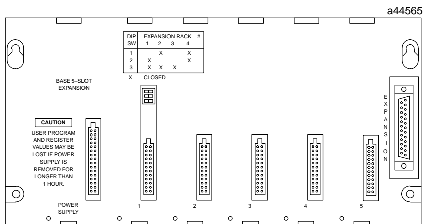
Figure 1-3. Exemple de platine d'extension Série 90-30 (modèle à 5 emplacements)
