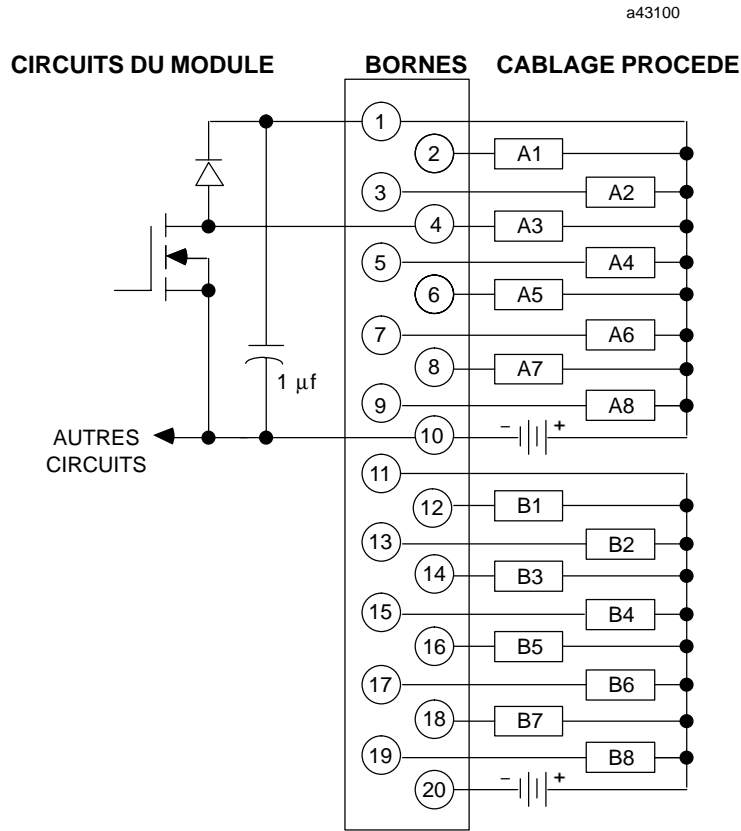
Figure 2-36. Câblage procédé - module de sortie logique négative 12/24 Vcc - 0,5 A - IC693MDL741
