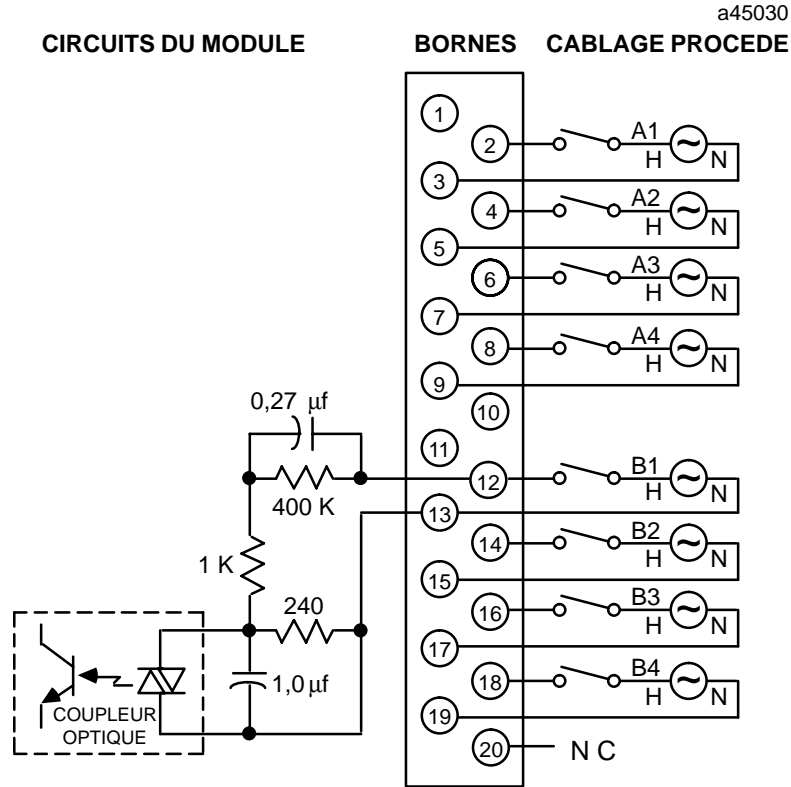
Figure 2-1. Câblage procédé - module d'entrée isolée 120 Vca - IC693MDL230
