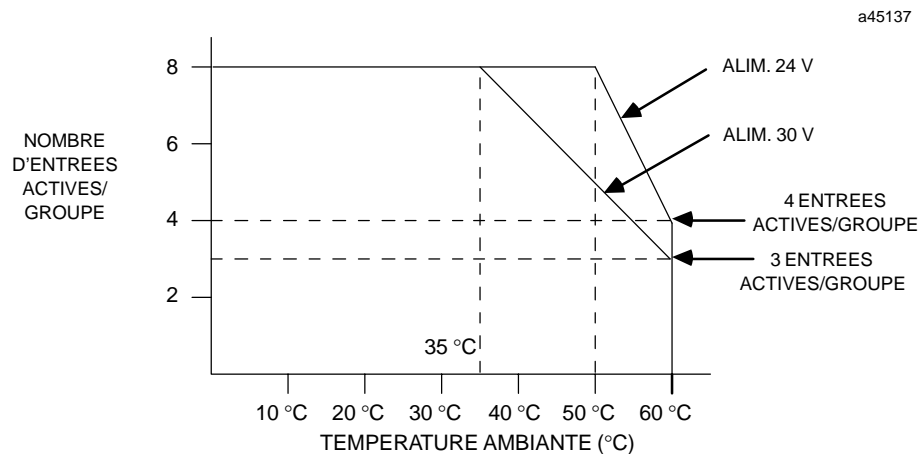
Figure 2-50. Points d'entrée du module IC694MDL655 suivant la température
