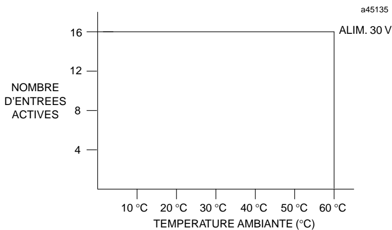
Figure 2-12. Points d'entrée du module IC693MDL645 suivant la température
