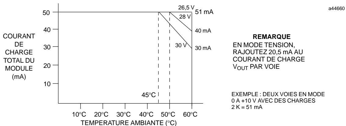
Figure 3-38. Déclassement du courant de charge
