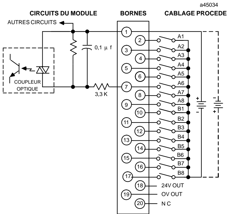
Figure 2-11. Câblage procédé - module d'entrée logique positive/négative 24 Vcc - IC693MDL645
