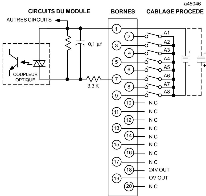
Figure 2-9. Câblage procédé - module d'entrée logique positive/négative 24 Vcc - IC693MDL634
