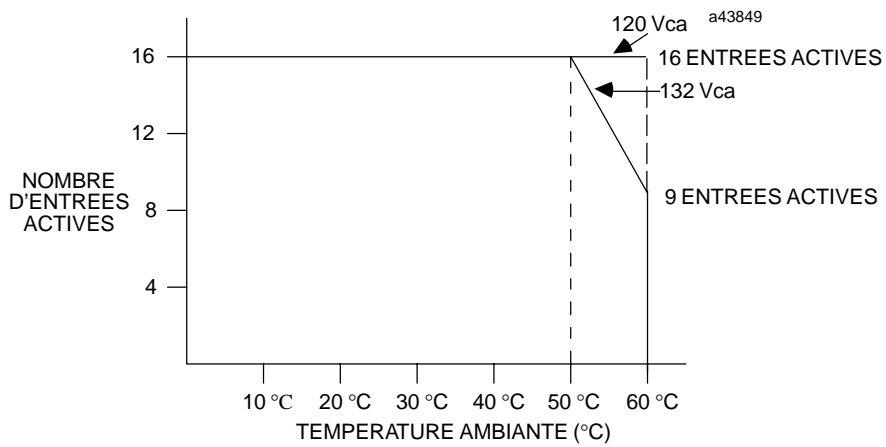
Figure 2-4. Points d'entrée du module IC693MDL240 suivant la température
