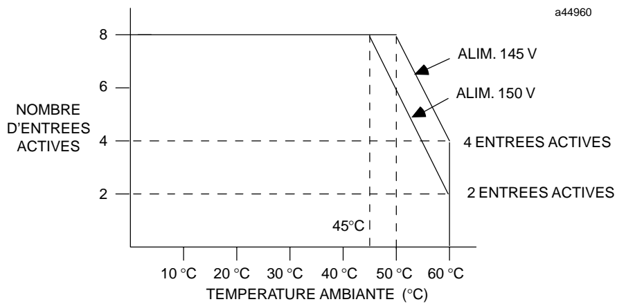
Figure 2-8. Points d'entrée du module IC693MDL632 suivant la température
