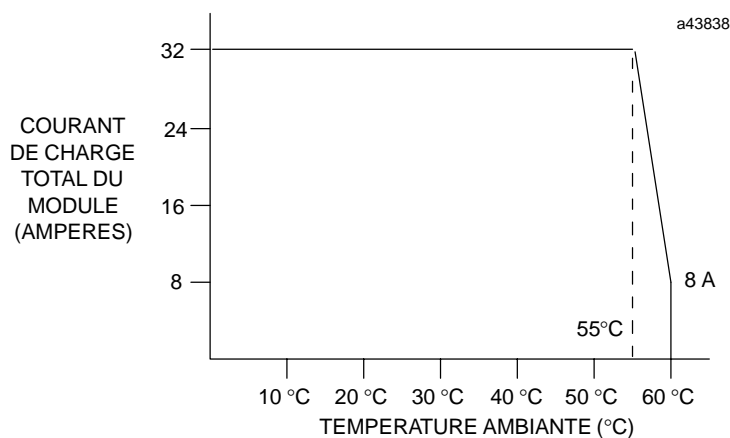
Figure 2-41. Courant de charge du module IC693MDL930 suivant la température
