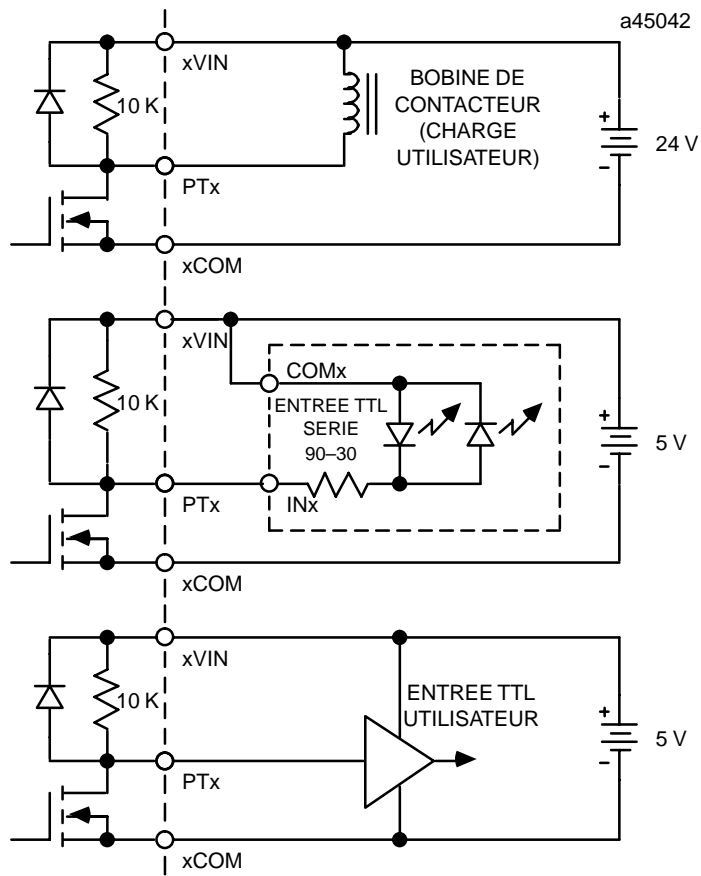
Figure 2-53. Exemples de raccordement aux charges utilisateur
