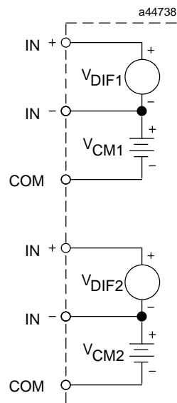
Figure 3-2. Tension de mode commun d'entrée analogique
