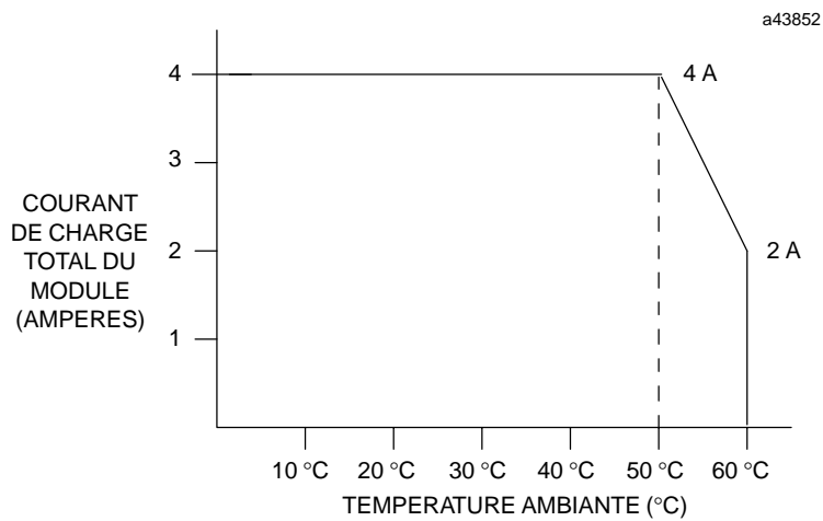
Figure 2-17. Points d'entrée du module IC693MDL310 suivant la température
