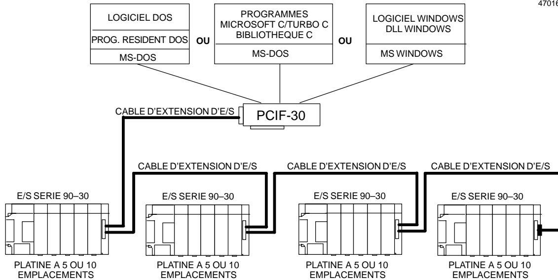
Figure 1-2. Exemple d'interface PCIF-30 vers le système d'E/S Série 90-30
