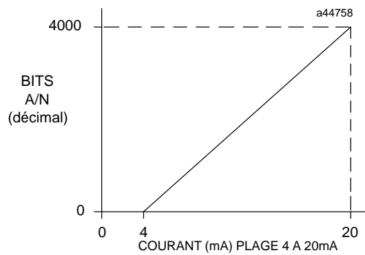
Figure 3-26. Bits A/N en fonction de l'entrée de courant pour le module IC693ALG223
