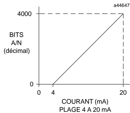
Figure 3-14. Bits A/N en fonction de l'entrée de courant, 4 à 20 mA
