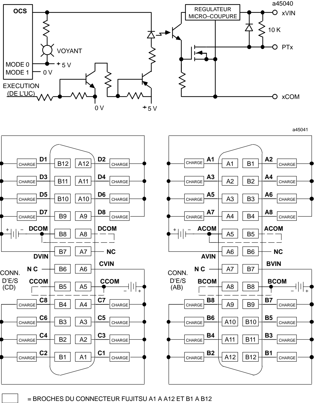
Figure 2-52. Câblage procédé - module de sortie 32 points logique négative 5/24 Vcc (TTL) - IC693MDL752
