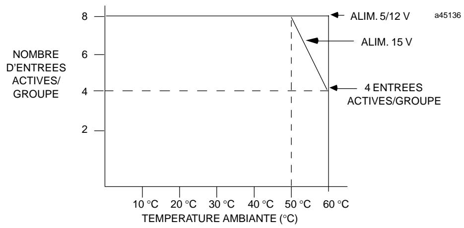
Figure 2-49. Points d'entrée du module IC693MDL654 suivant la température
