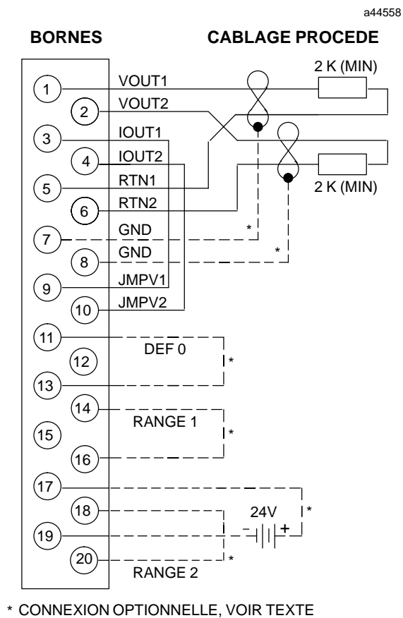
Figure 3-41. Câblage procédé - module de sortie de courant analogique (mode tension) - IC693ALG391
