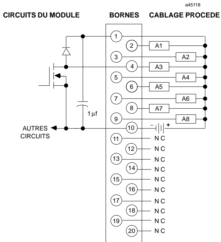
Figure 2-30. Câblage procédé - module de sortie logique négative 12/24 Vcc - 0,5 A - IC693MDL733
