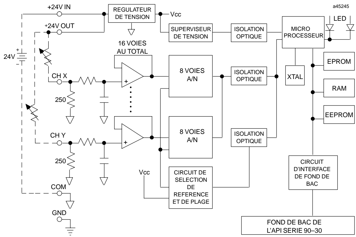
Figure 3-27. Schéma fonctionnel du module d'entrée de courant analogique 16 voies - IC693ALG223
