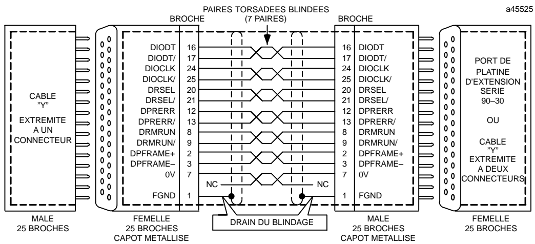
Figure C-1. Schéma de câblage point-à-point pour les câbles de longueur personnalisée
