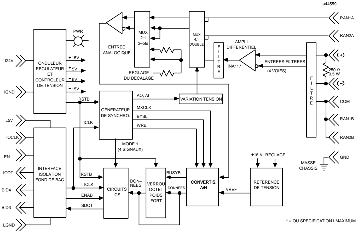
Figure 3-18. Schéma fonctionnel du module d'entrée de courant analogique - IC693ALG221
