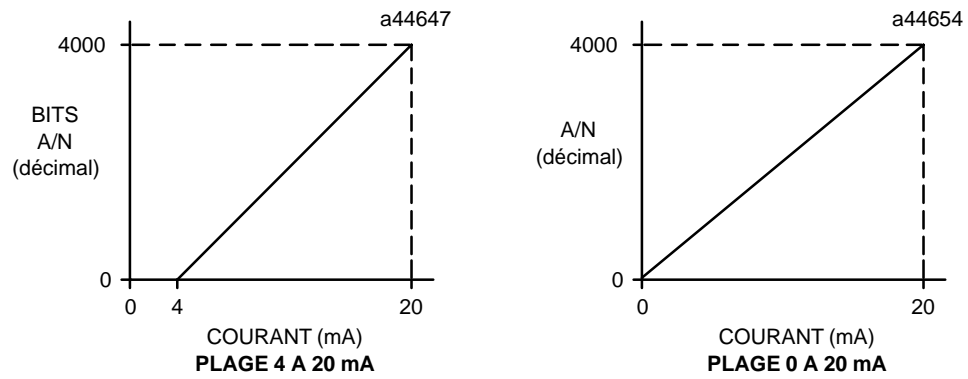
Figure 3-48. Bits A/N en fonction de l'entrée courant
