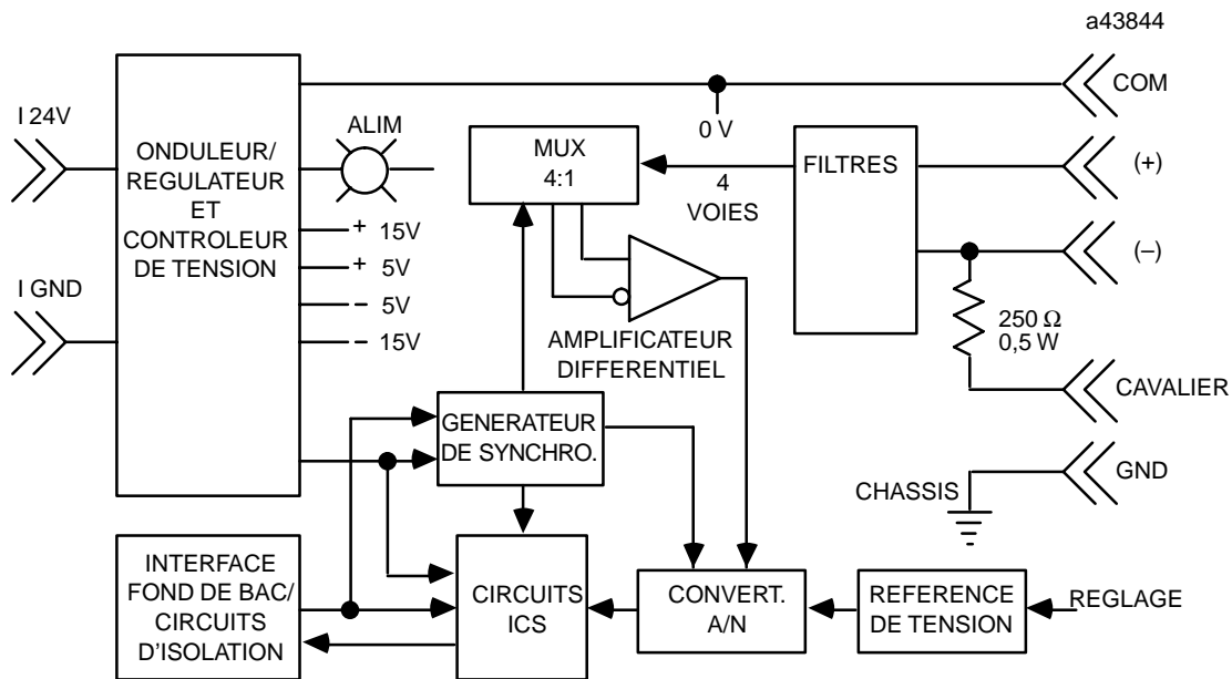
Figure 3-12. Schéma fonctionnel du module d'entrée de tension analogique, IC693ALG220
