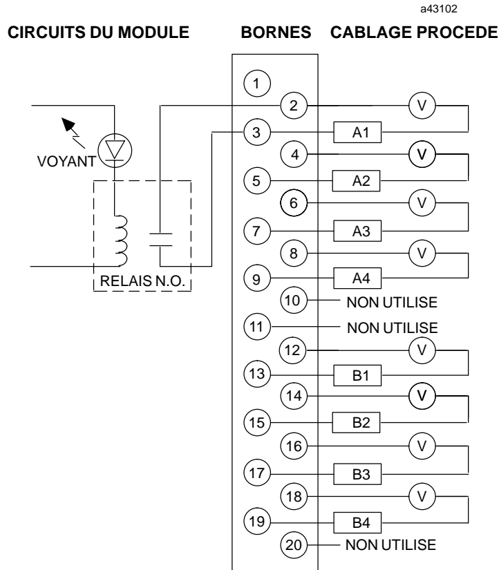
Figure 2-40. Câblage procédé - module de sortie à relais isolée 4 A - IC693MDL930
