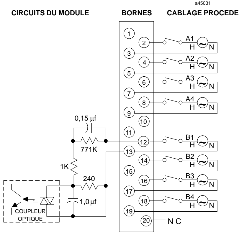
Figure 2-2. Câblage procédé - module d'entrée isolée 240 Vca - IC693MDL231
