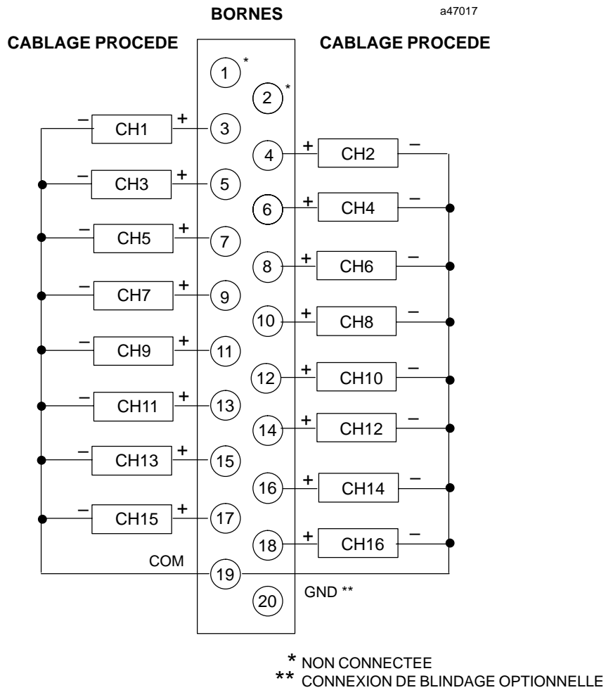
Figure 3-23. Câblage procédé du module d'entrée de tension analogique 16 voies - IC693ALG222 (Mode non référencé)
