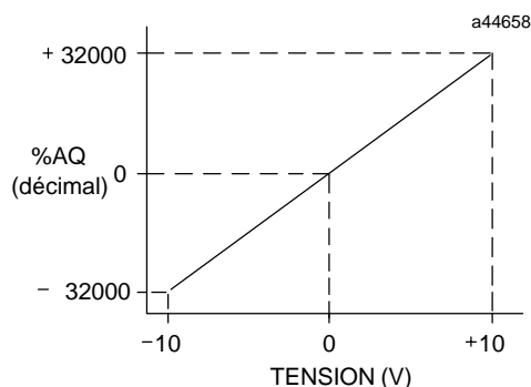
Figure 3-31. Mise à l'échelle de la sortie de tension
