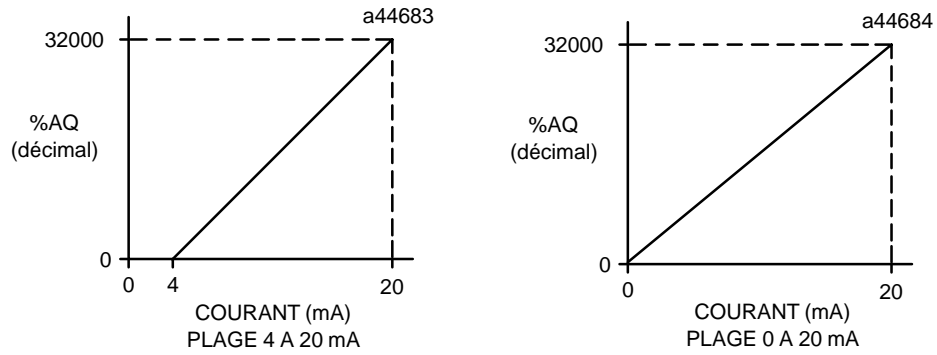
Figure 3-50. Mise à l'échelle de la sortie courant
