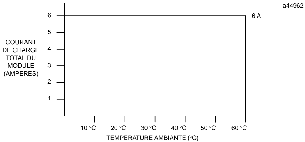
Figure 2-21. Courant de charge du module IC693MDL340 suivant la température
