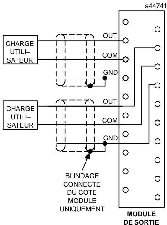
Figure 3-9. Connexion du blindage pour les modules de sortie analogiques
