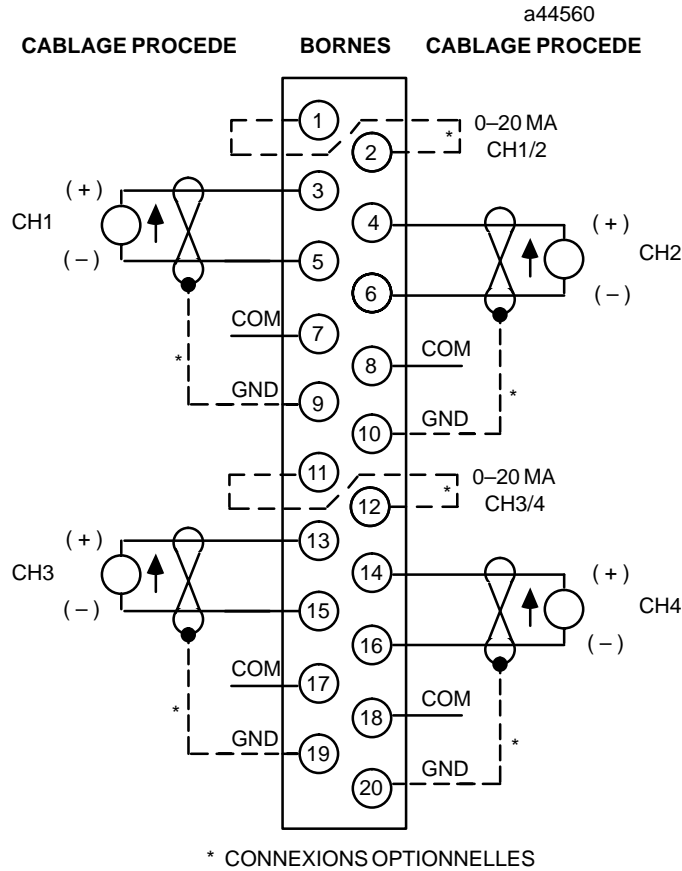
Figure 3-19. Câblage procédé du module d'entrée de courant analogique 4 voies
