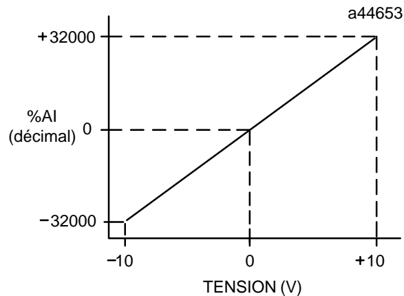
Figure 3-11. Mise à l'échelle de l'entrée de tension
