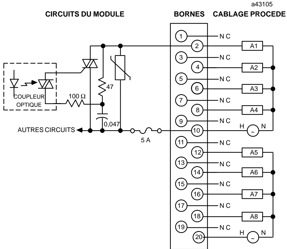
Figure 2-18. Câblage procédé - module de sortie 120/240 Vca - 2 A - IC693MDL330
