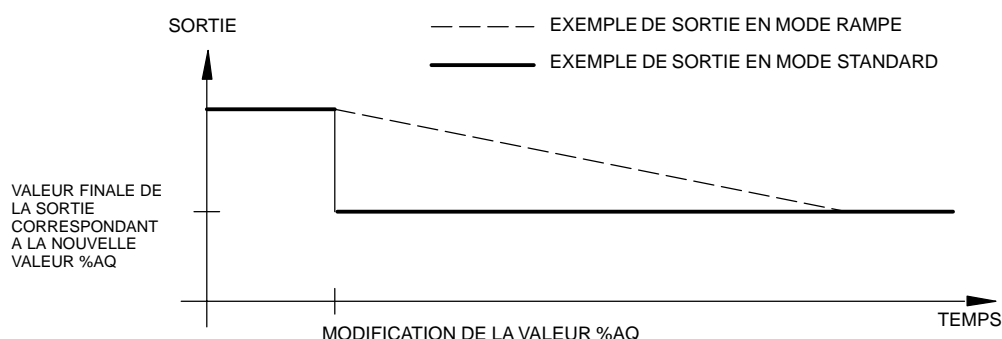
Figure 3-52. Comportement de la sortie en mode Rampe et en mode Standard
