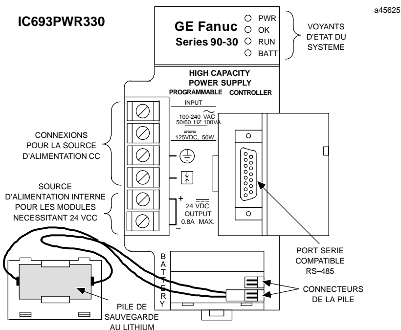
Figure 1-19. Alimentation haute capacité d'entrée CA/CC - IC693PWR330
