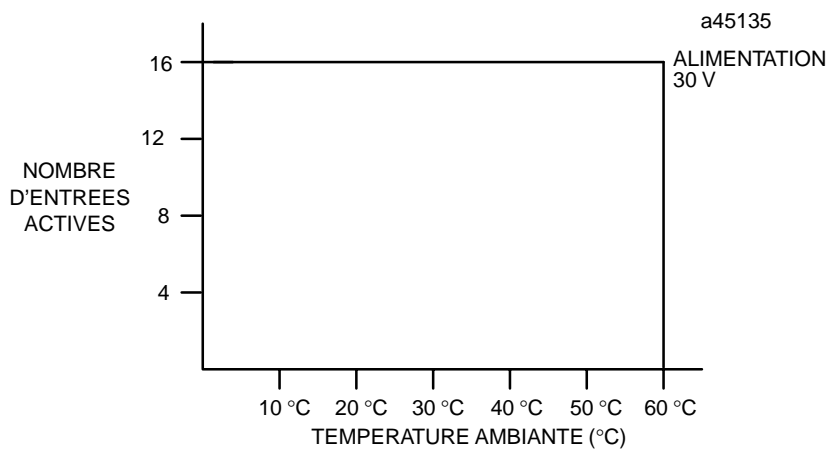
Figure 2-6. Points d'entrée du module IC693MDL241 suivant la température
