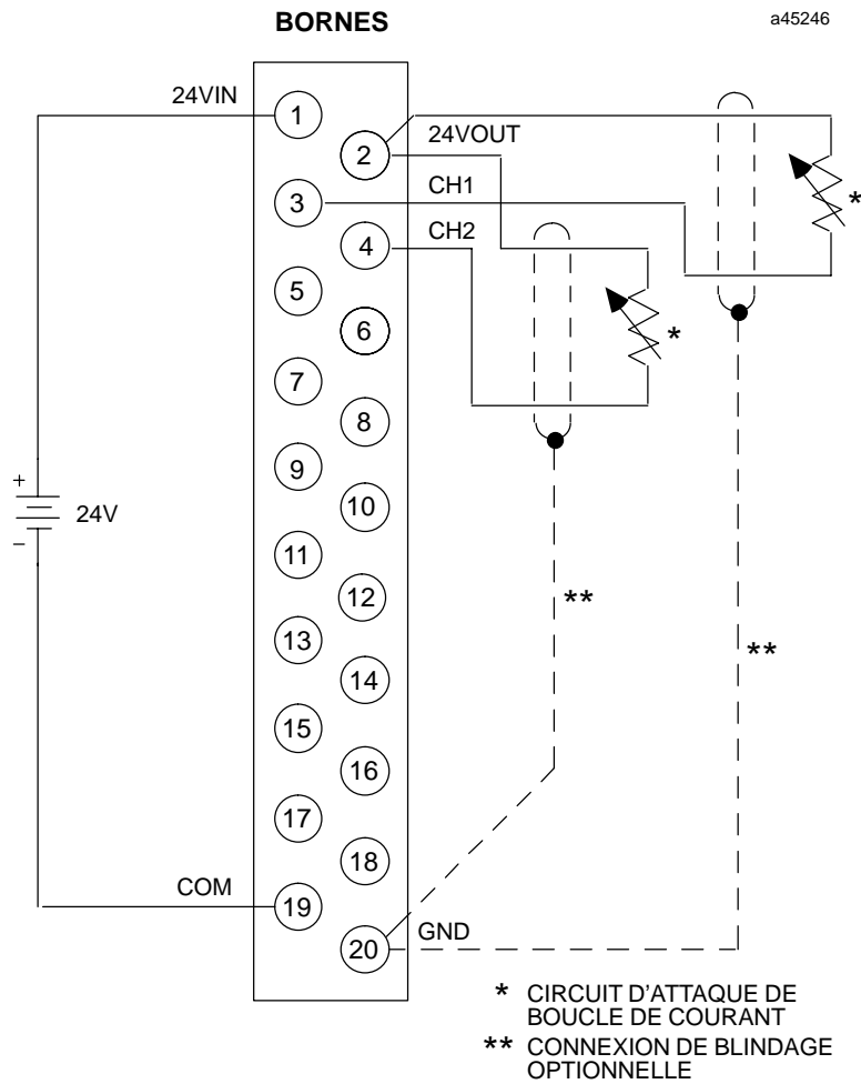
Figure 3-28. Câblage procédé du module d'entrée de courant analogique 16 voies - IC693ALG223
