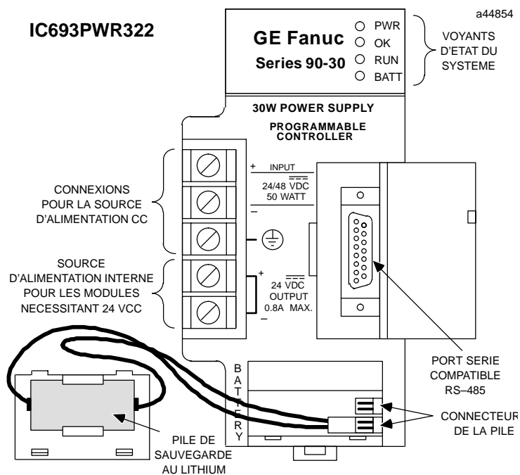
Figure 1-21. Alimentation d'entrée CC du 90-30 – IC693PWR322
