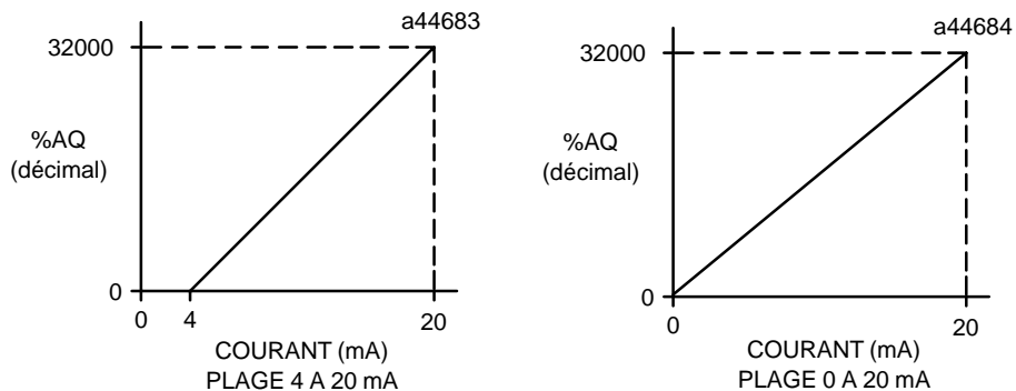
Figure 3-42. Mise à l'échelle de la sortie courant
