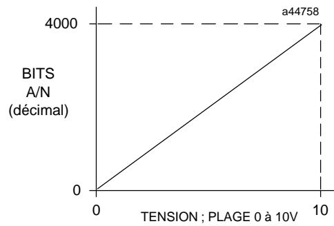
Figure 3-21. Bits A/N en fonction de l'entrée de tension pour le module IC693ALG222
