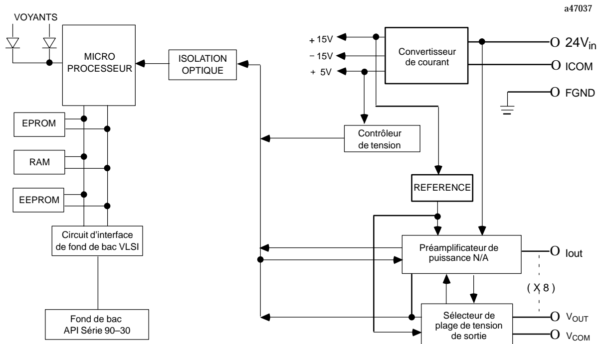
Figure 3-46. Schéma fonctionnel du module IC693ALG392
