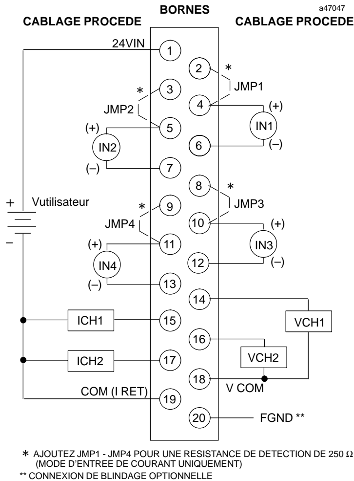
Figure 3-54. Câblage procédé du module analogique mixte - IC693ALG442
