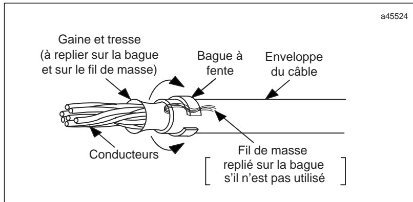
Figure 1-11. Utilisation de la bague à fente avec la gaine et la tresse du blindage
