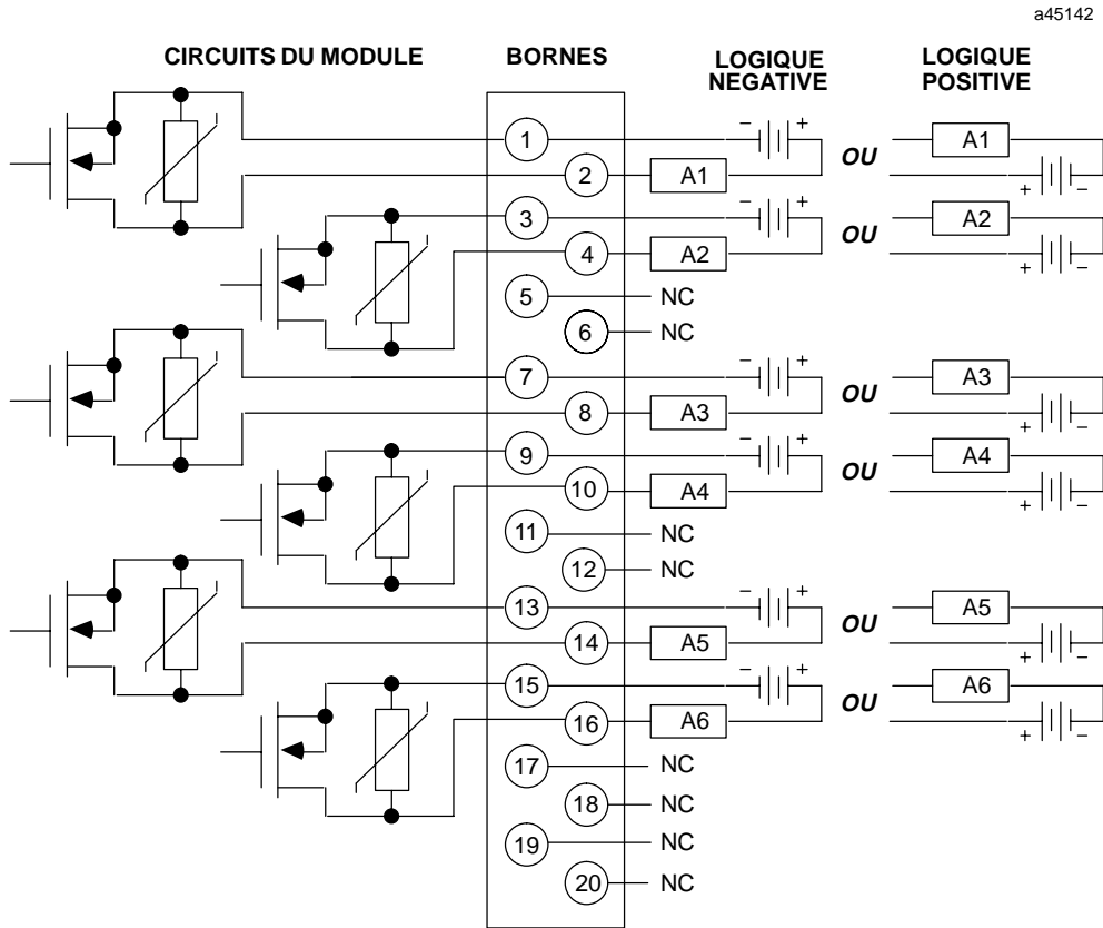
Figure 2-32. Câblage procédé - module de sortie logique positive/négative 125 Vcc - 1 A - IC697MDL734
