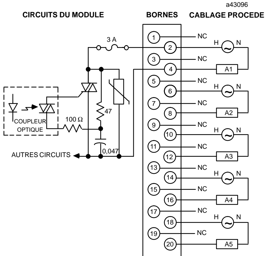
Figure 2-22. Câblage procédé - module de sortie isolée 120/240 Vca - IC693MDL390
