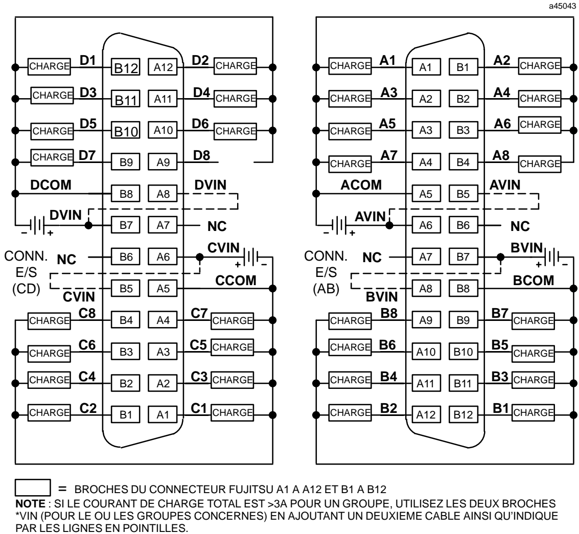
Figure 2-54. Câblage procédé - module de sortie 32 points logique positive 12/24 Vcc - 0,5 A - IC693MDL753
