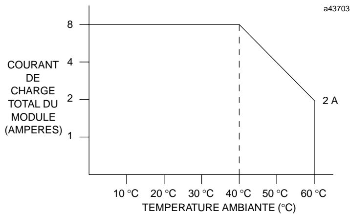
Figure 2-19. Points d'entrée du module IC693MDL330 suivant la température
