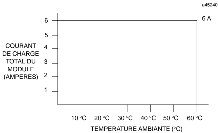
Figure 2-33. Courant de charge du module IC697MDL734 suivant la température
