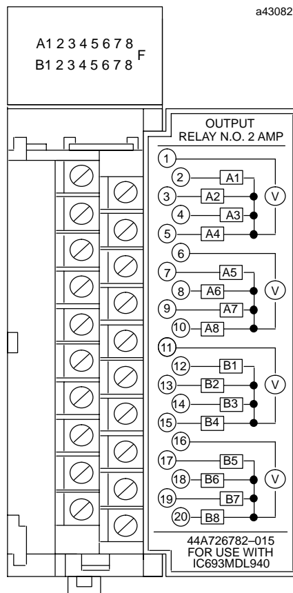
Figure 1-1. Exemple de module d'E/S Série 90-30
