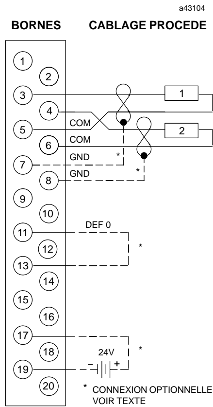
Figure 3-33. Câblage procédé du module de sortie de tension analogique - IC693ALG390
