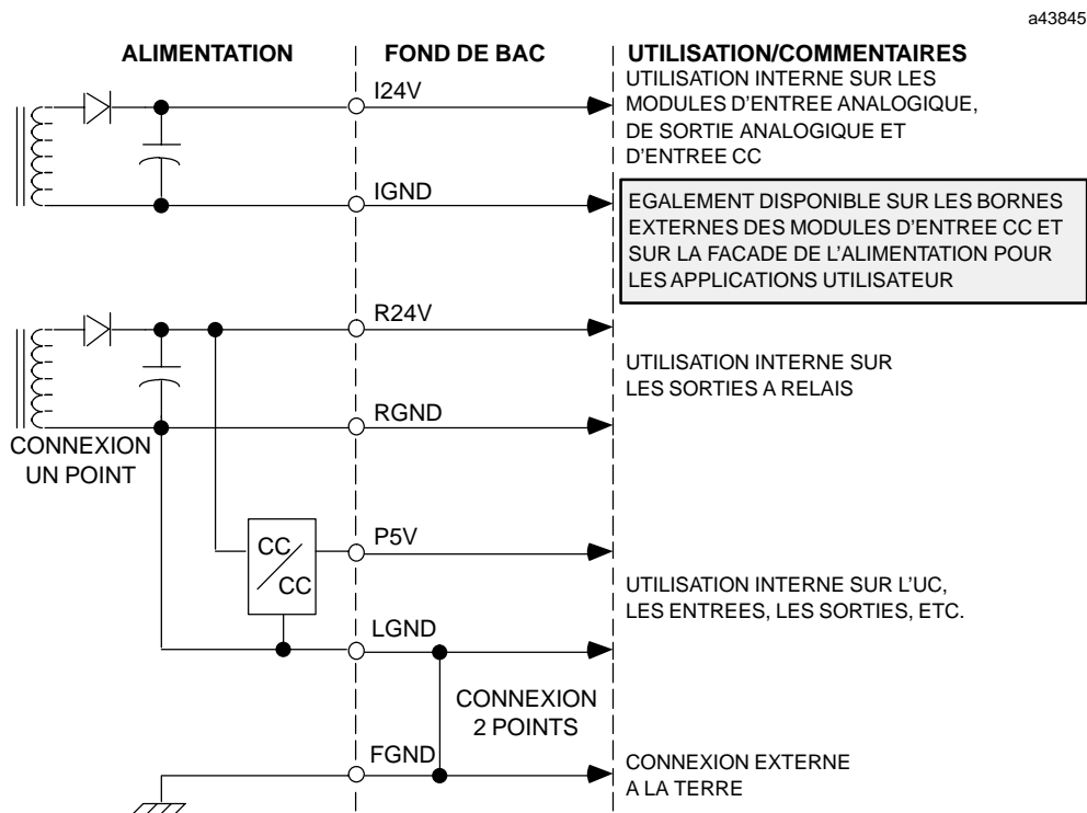
Figure 1-18. Interconnexion d'alimentations
