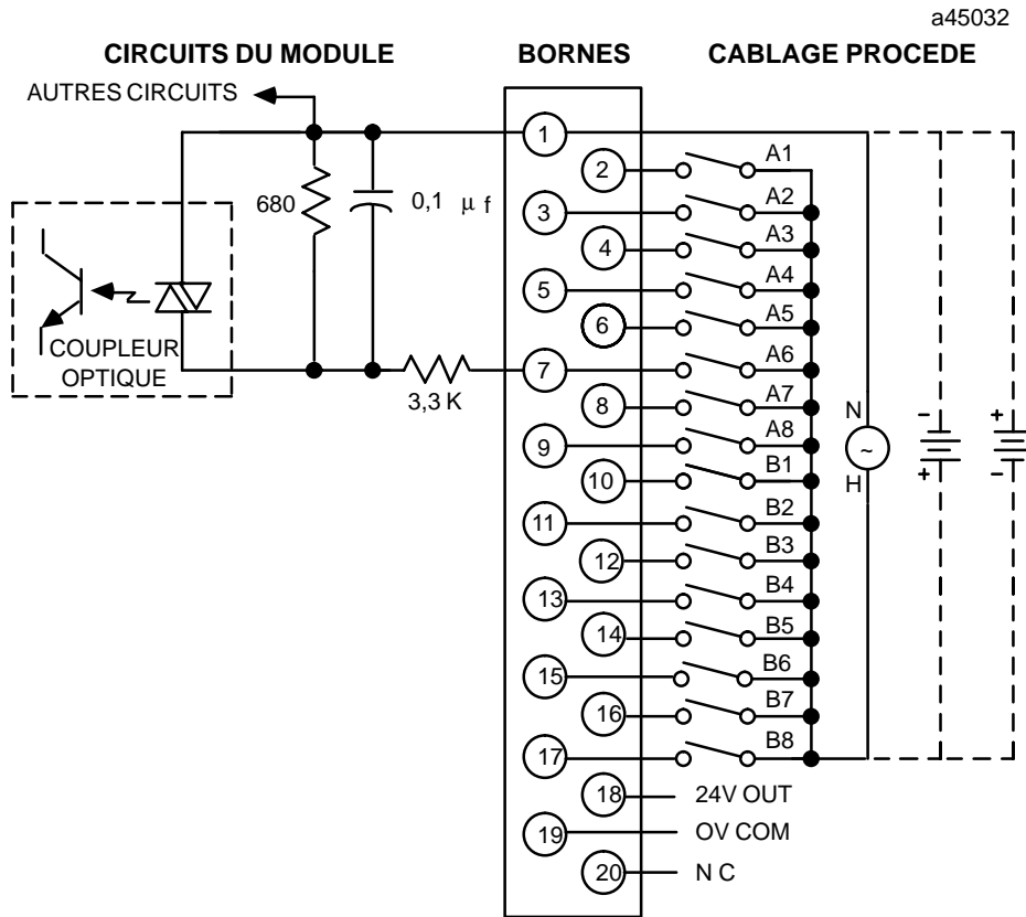
Figure 2-5. Câblage procédé - module d'entrée logique positive/négative 24 volts CA/CC - IC693MDL241
