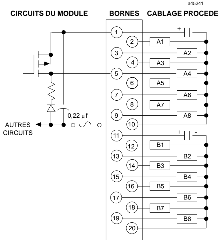
Figure 2-38. Câblage procédé - module de sortie logique positive 12/24 Vcc - 1 A - ESCP - IC693MDL742
