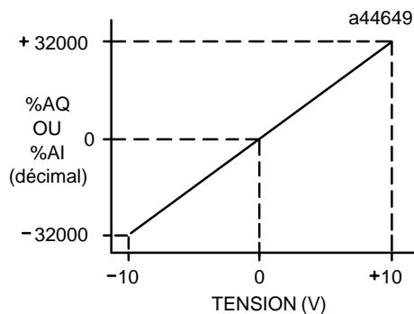
Figure 3-6. Tension en fonction du mot de donnée
