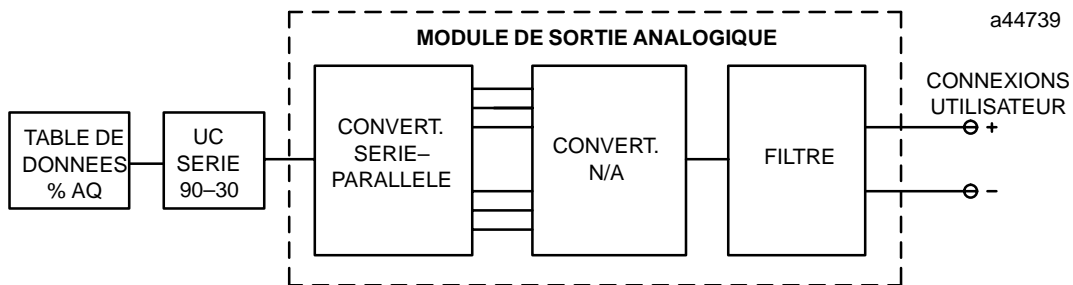
Figure 3-3. Schéma fonctionnel d'une sortie analogique
