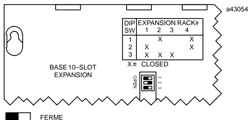
Figure 1-9. Exemple de configuration de numéro de bac (bac numéro 2 sélectionné)
