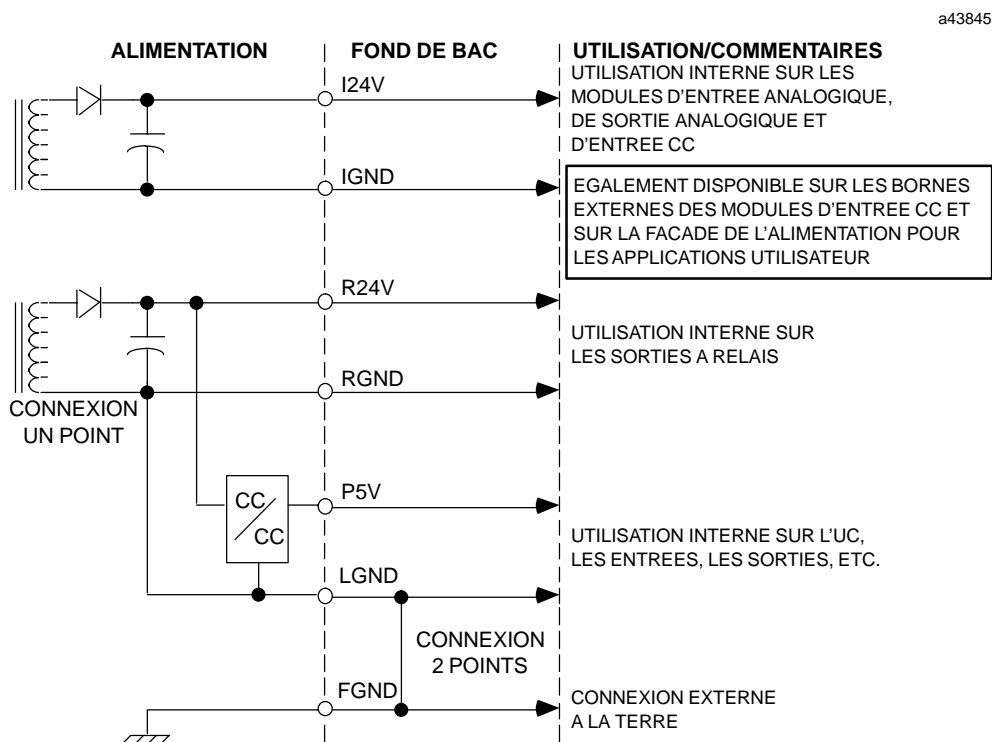
Figure 1-16. Interconnexion d'alimentations
