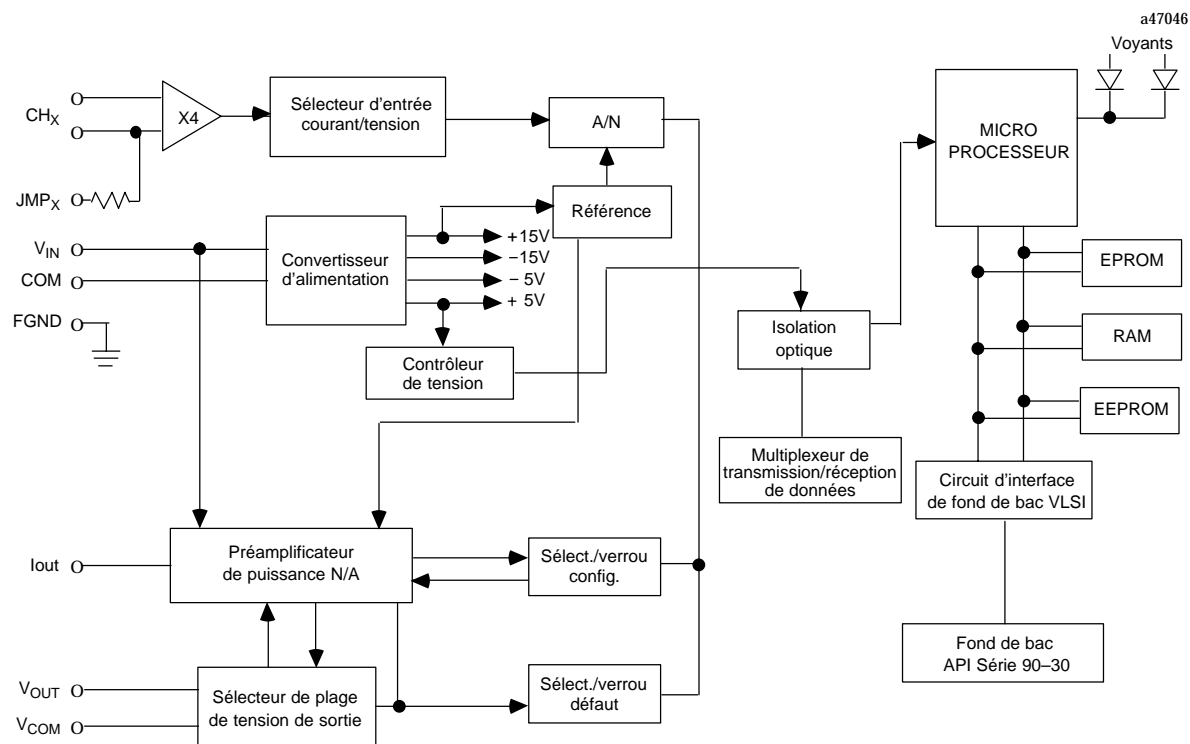
Figure 3-53. Schéma fonctionnel du module analogique mixte - IC693ALG442
