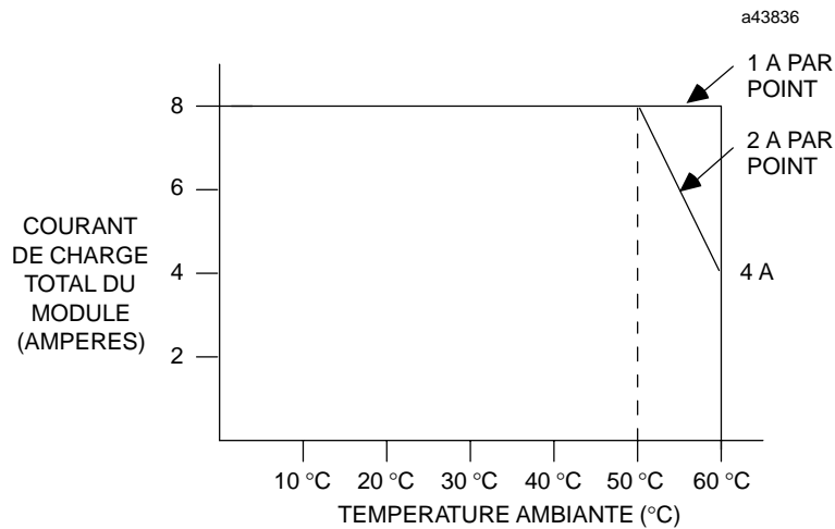
Figure 2-25. Courant de charge du module IC693MDL730 suivant la température
