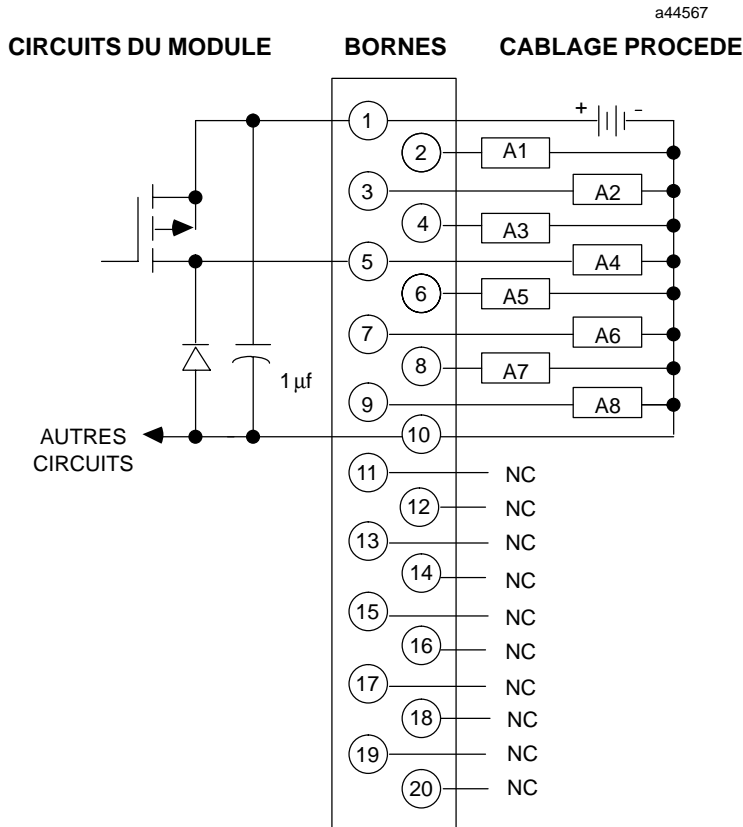
Figure 2-28. Câblage procédé - module de sortie logique positive 12/24 Vcc - 0,5 A - IC693MDL732
