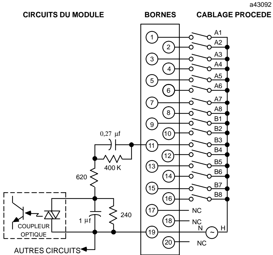
Figure 2-3. Câblage procédé - module d'entrée 120 Vca - IC693MDL240
