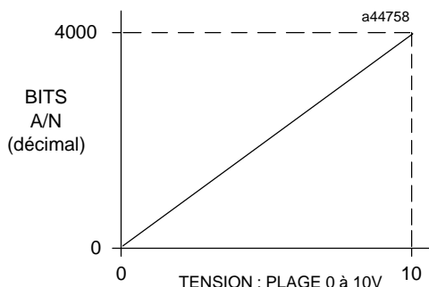
Figure 3-49. Bits A/N en fonction de l'entrée tension
