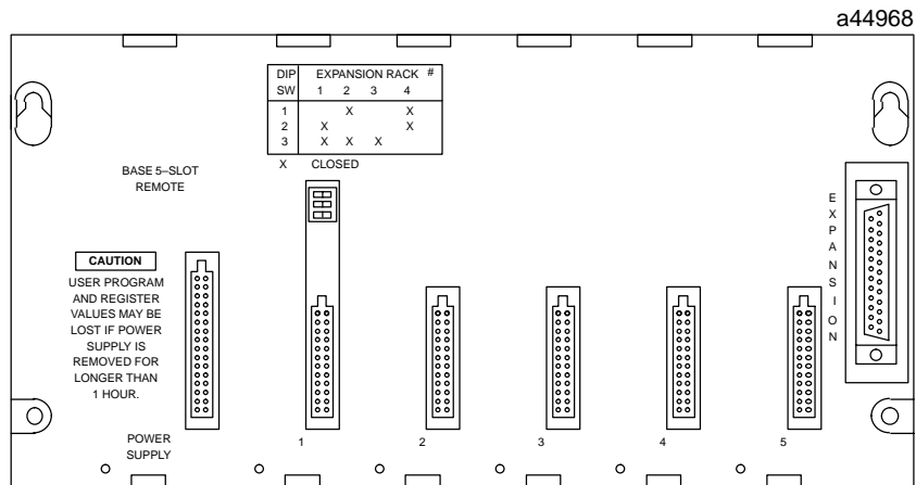
Figure 1-4. Exemple de platine déportée Série 90-30 (modèle à 5 emplacements)
