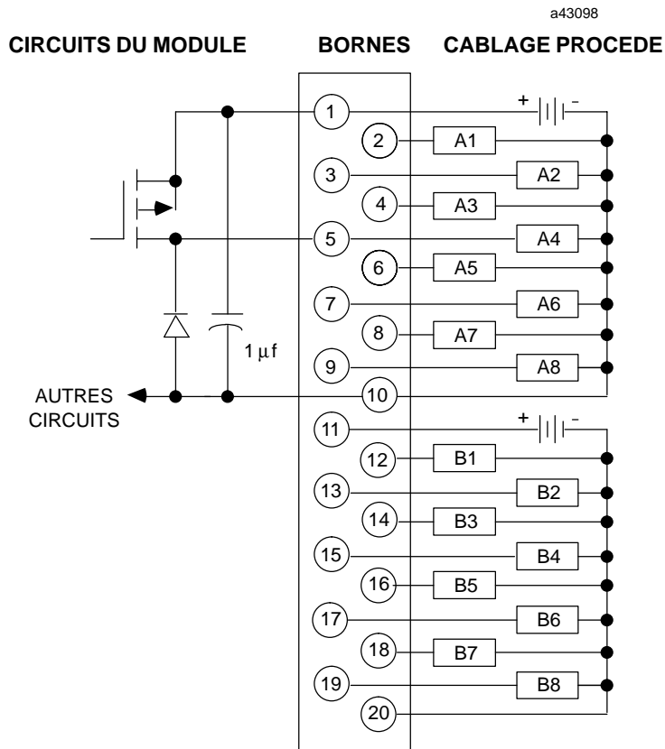
Figure 2-34. Câblage procédé - module de sortie logique positive 12/24 Vcc - 0,5 A - IC693MDL740
