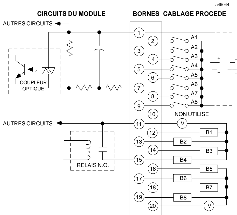
Figure 2-47. Câblage procédé - module d'entrée 24 Vcc/sortie à relais - IC693MDR390
