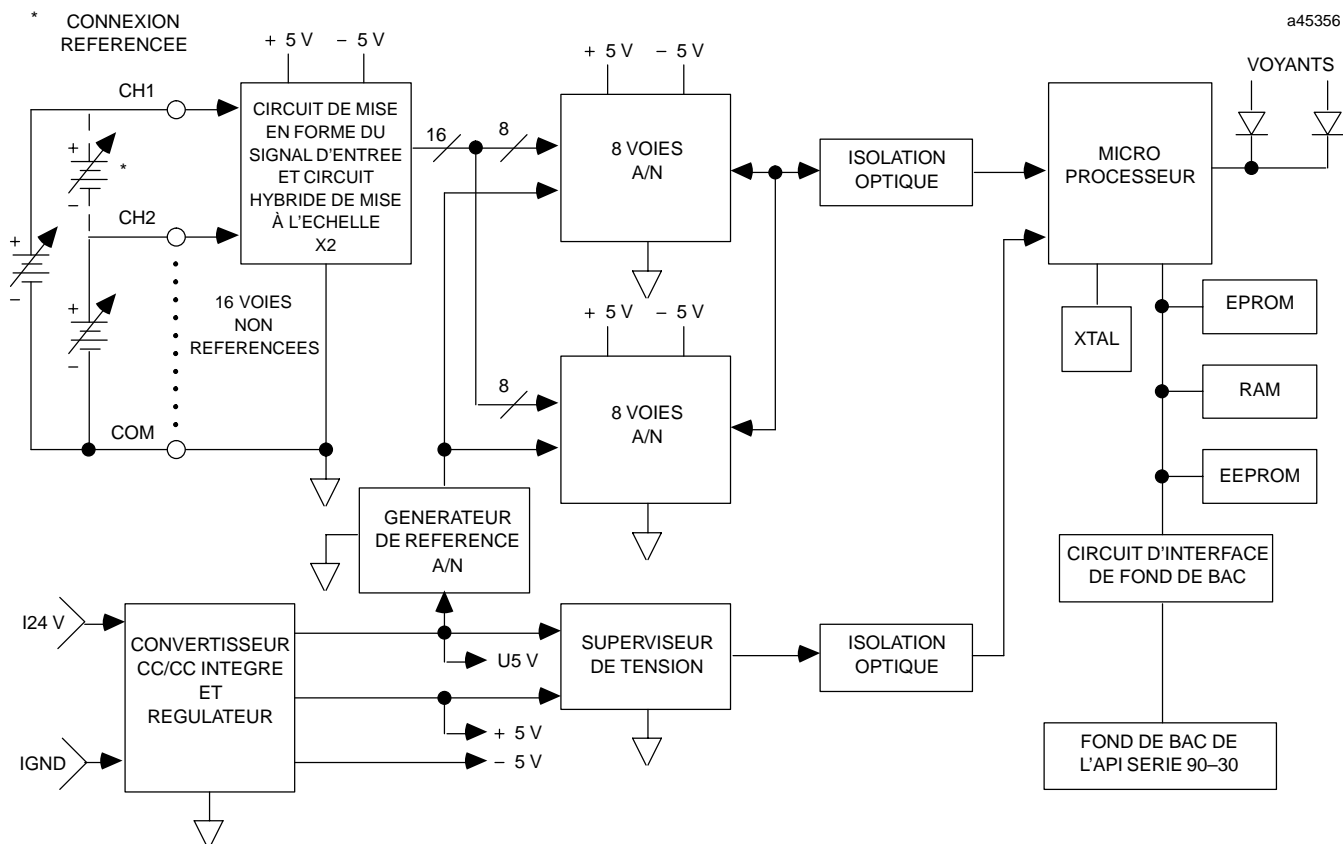
Figure 3-22. Schéma fonctionnel du module d'entrée de tension analogique 16 voies - IC693ALG222
