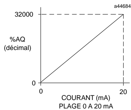
Figure 3-37. Mise à l'échelle de la sortie de courant, 0 à 20 mA
