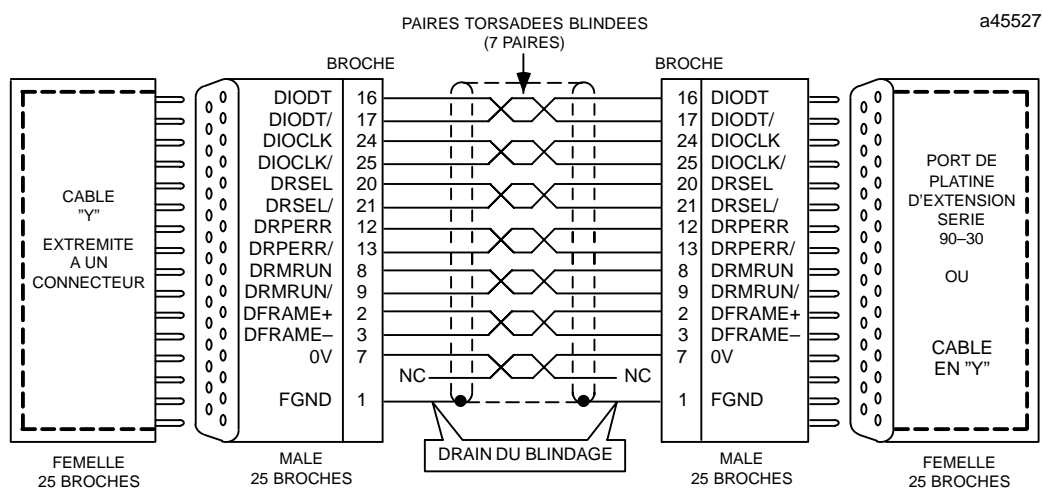
Figure 1-14. Schéma de câblage point-à-point pour les applications industrielles habituelles
