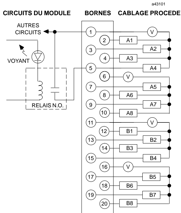
Figure 2-44. Câblage procédé - module de sortie à relais N.O. - 2 A - IC693MDL940
