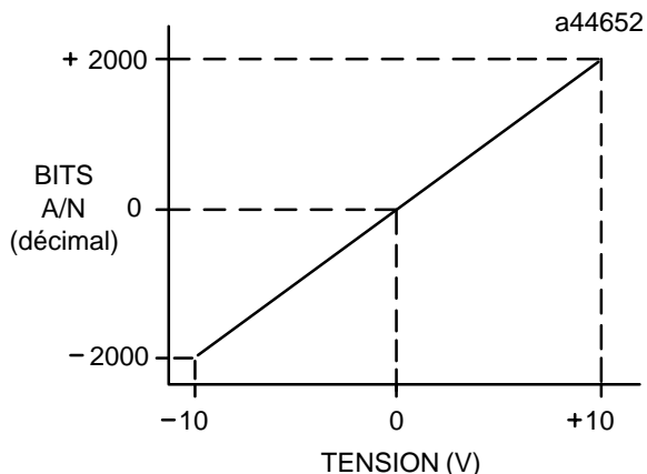
Figure 3-10. Bits A/N en fonction de l'entrée de tension
