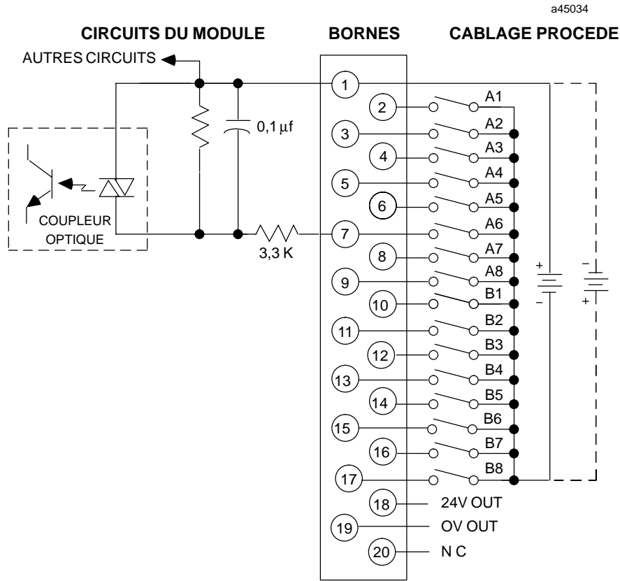
Figure 2-13. Câblage procédé - module d'entrée logique positive/négative 24 Vcc rapide - IC693MDL646
