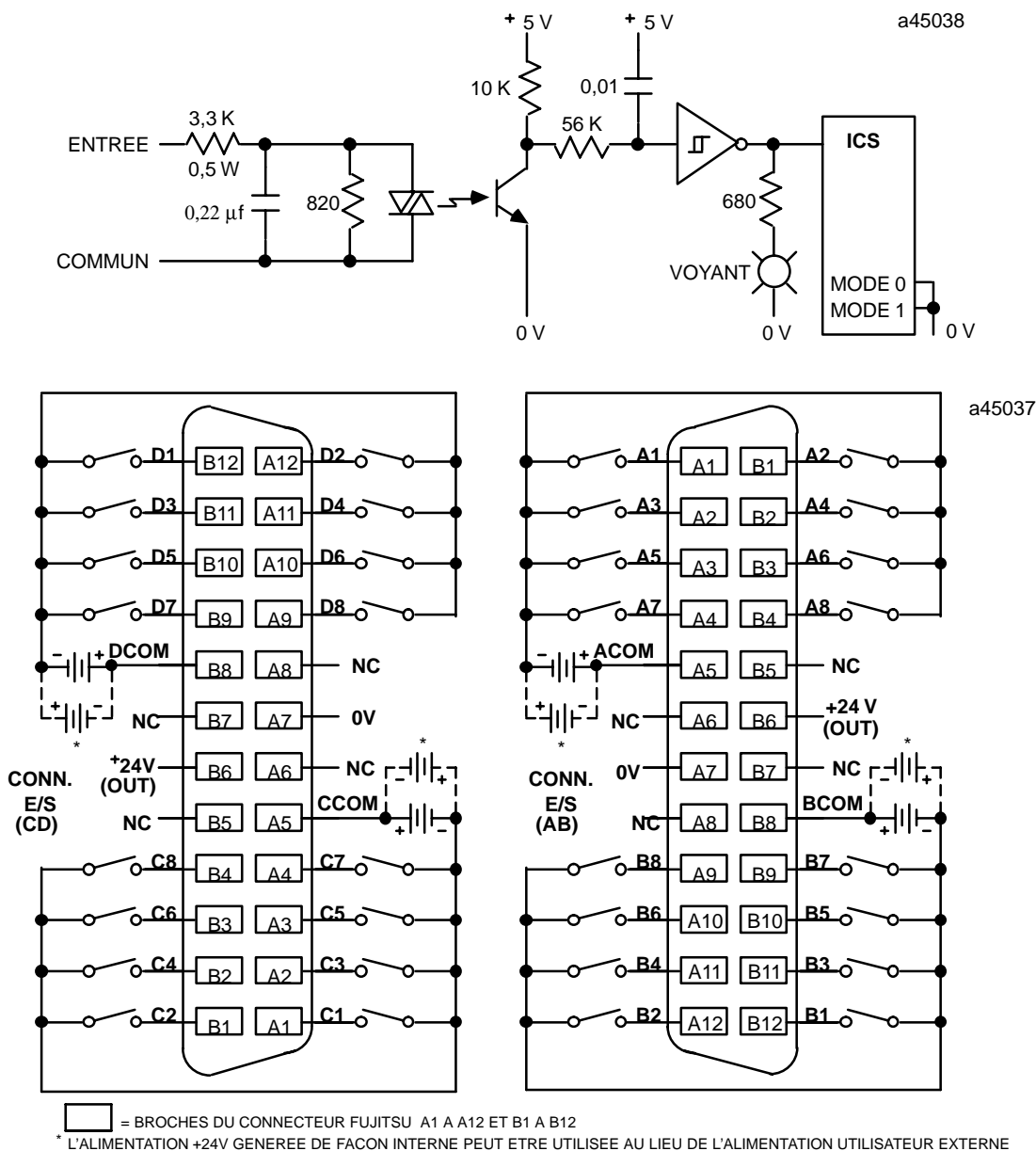
Figure 2-51. Câblage procédé - module d'entrée 32 points logique positive/négative 24 Vcc - IC693MDL655
