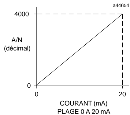
Figure 3-15. Bits A/N en fonction de l'entrée de courant, 0 à 20 mA
