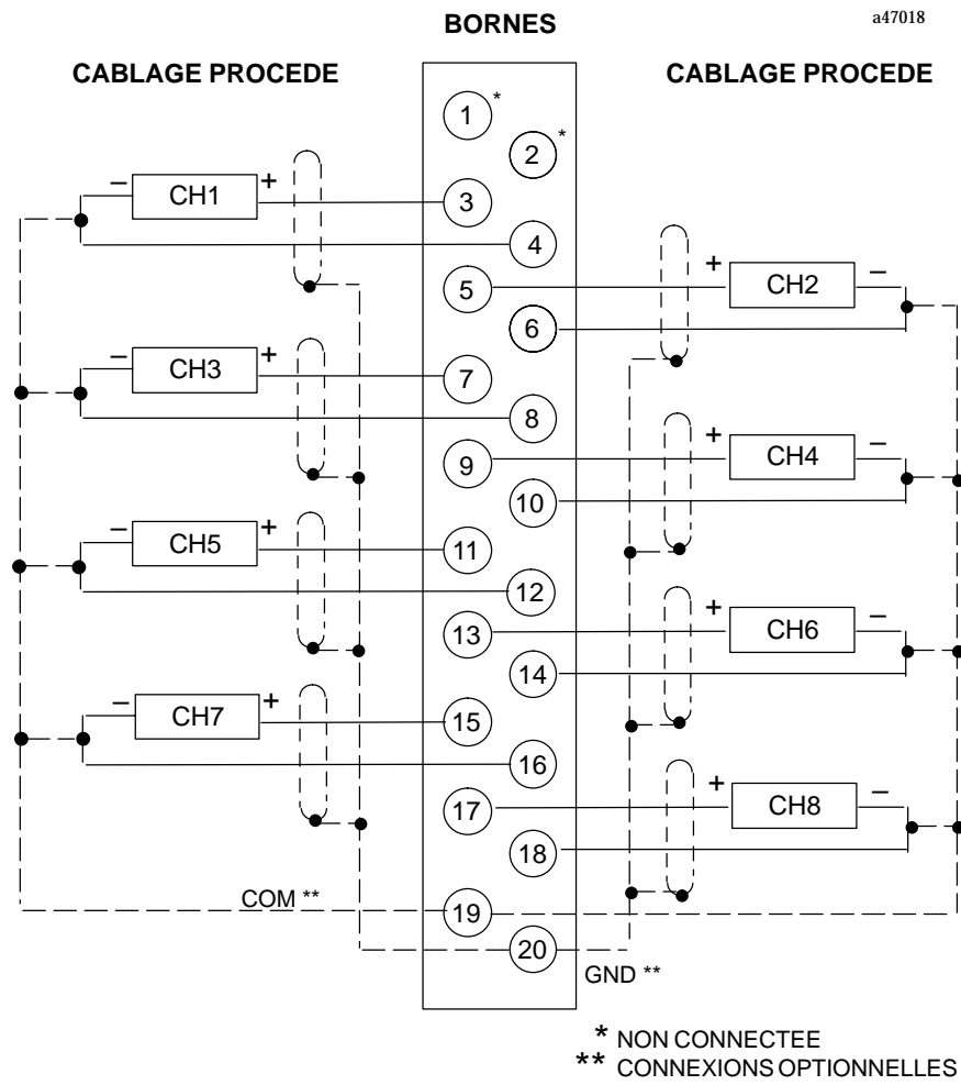
Figure 3-24. Câblage procédé du module d'entrée de tension analogique 16 voies - IC693ALG222 (Mode référencé)
