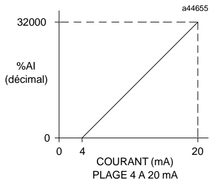
Figure 3-16. Mise à l'échelle du module d'entrée de courant analogique, 4 à 20 mA
