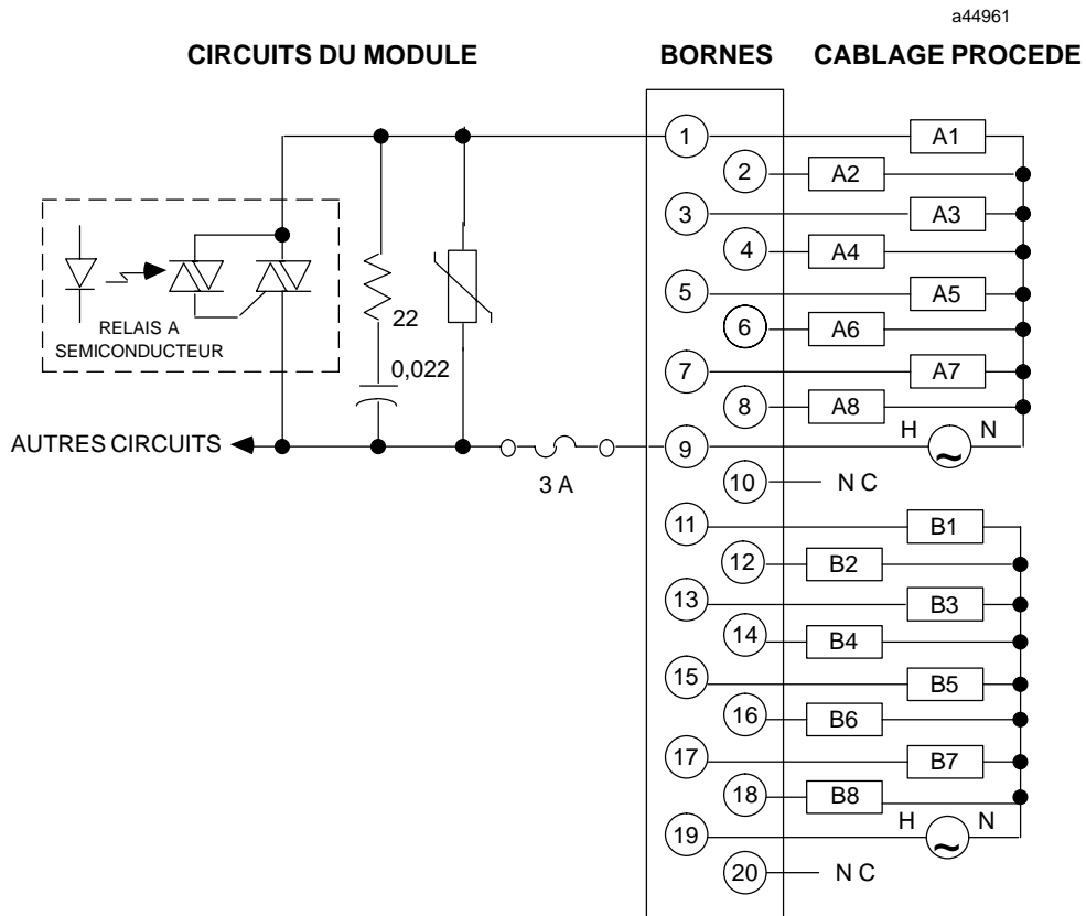
Figure 2-20. Câblage procédé - module de sortie 120 Vca - 0,5 A - IC693MDL340
