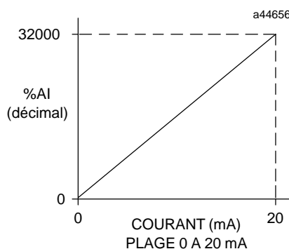
Figure 3-17. Mise à l'échelle du module d'entrée de courant analogique, 0 à 20 mA
