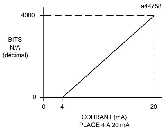
Figure 3-4. Bits N/A en fonction de la sortie de courant pour le module IC693ALG391
