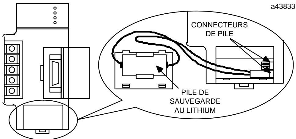
Figure 1-25. Pile de sauvegarde pour mémoire RAM
