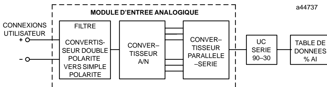
Figure 3-1. Schéma fonctionnel d'une entrée analogique
