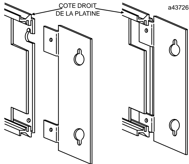
Figure 1-7. Installation du support de montage de platine
