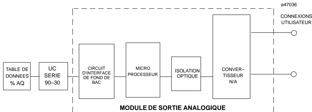
Figure 3-44. Schéma fonctionnel du module IC693ALG392
