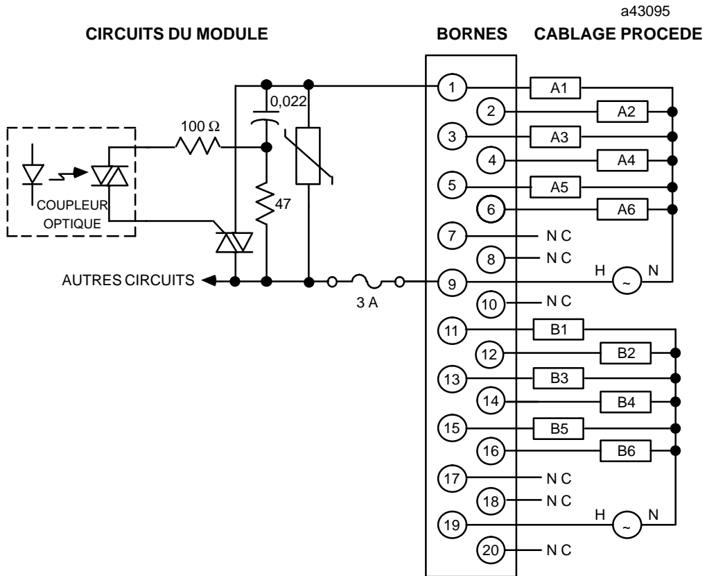
Figure 2-16. Câblage procédé - module de sortie 120 Vca - 0,5 A - IC693MDL310
