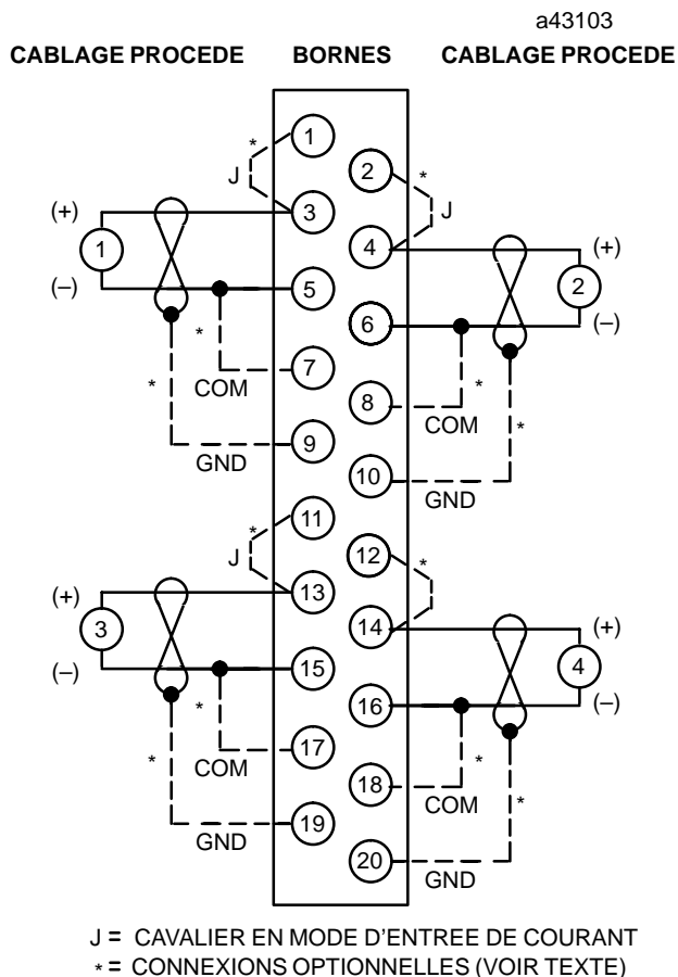
Figure 3-13. Câblage procédé du module d'entrée de tension analogique 4 voies
