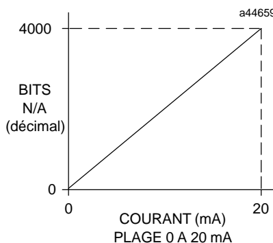
Figure 3-35. Bits N/A en fonction de la sortie de courant, 0 à 20 mA
