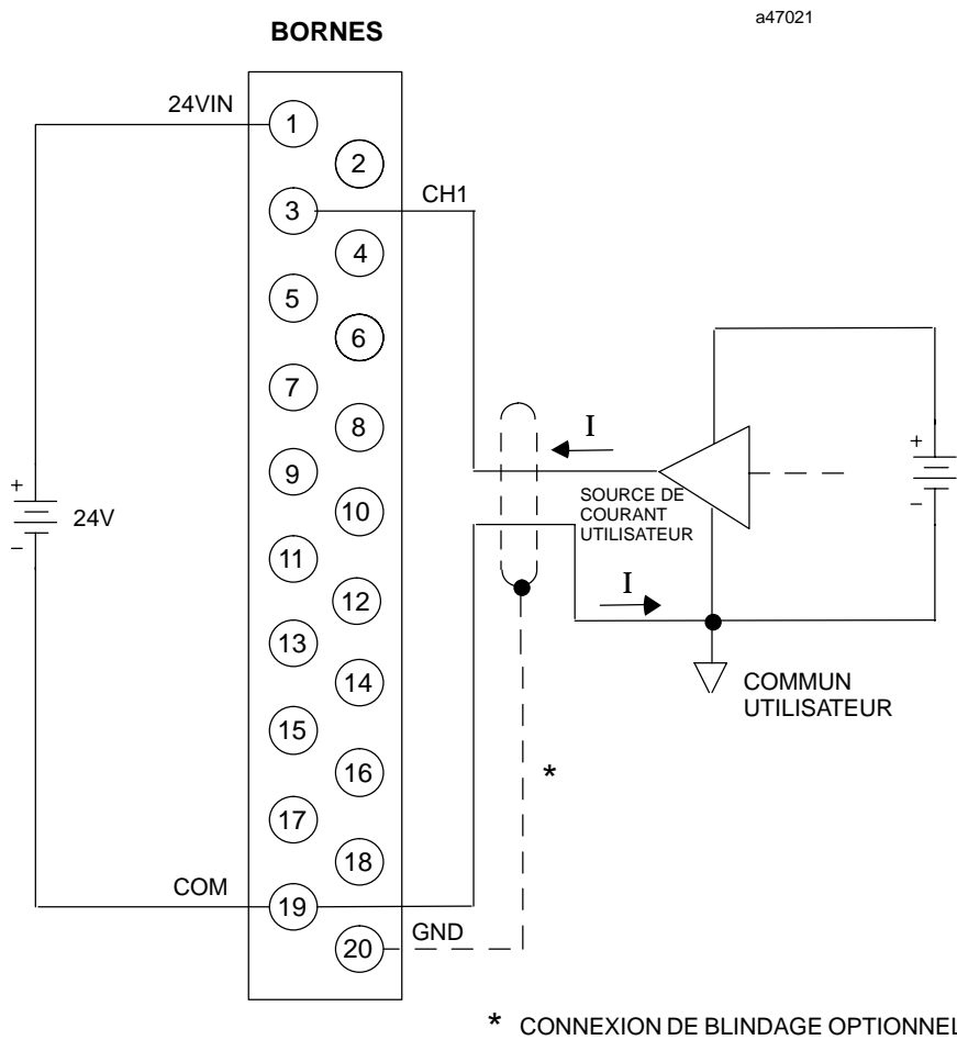
Figure 3-29. Câblage procédé - Autres connexions utilisateur - IC693ALG223
