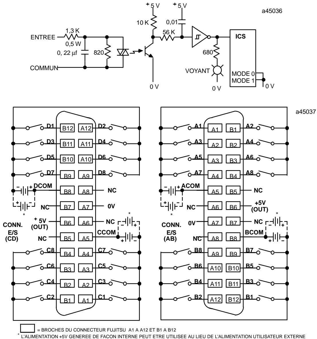
Figure 2-48. Câblage procédé - module d'entrée 32 points logique positive/négative 5/12 Vcc (TTL) - IC693MDL654
