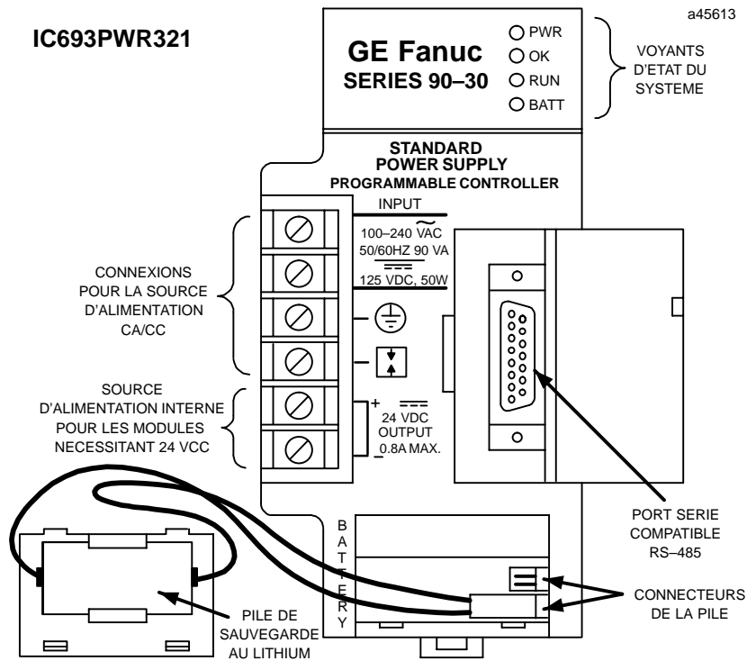
Figure 1-17. Alimentation standard d'entrée CA/CC du 90-30 – IC693PWR321
