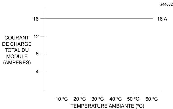
Figure 2-45. Courant de charge du module IC693MDL940 suivant la température
