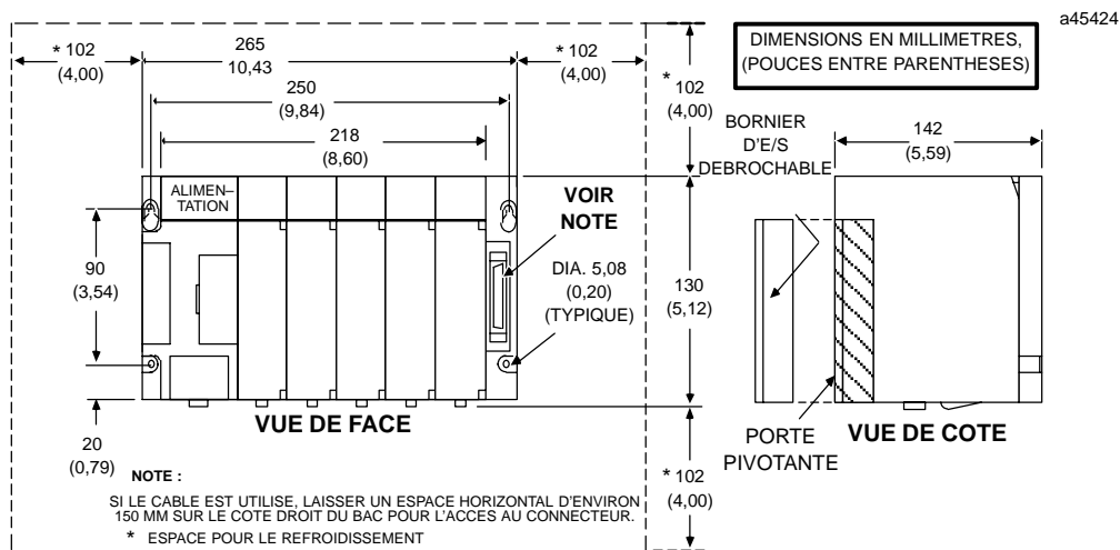
Figure 1-5. Dimensions de montage et espace nécessaire pour les platines à 5 emplacements
