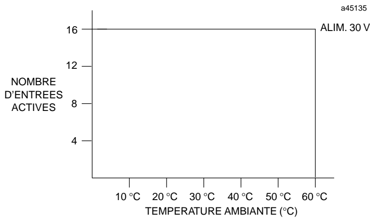
Figure 2-14. Points d'entrée du module IC693MDL646 suivant la température
