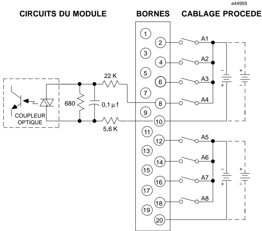
Figure 2-7. Câblage procédé - module d'entrée logique positive/négative 125 Vcc - IC693MDL632
