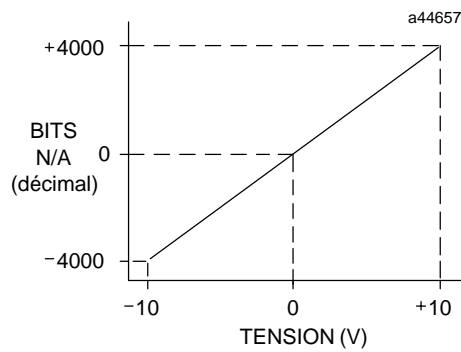
Figure 3-30. Bits N/A en fonction de la sortie de tension
