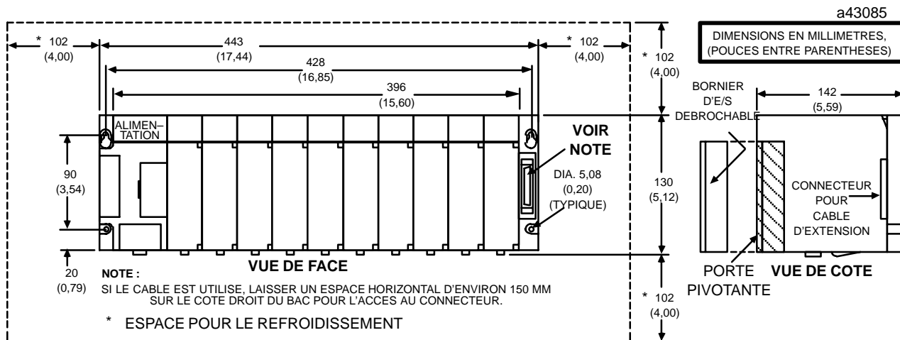
Figure 1-6. Dimensions de montage et espace nécessaire pour les platines à 10 emplacements
