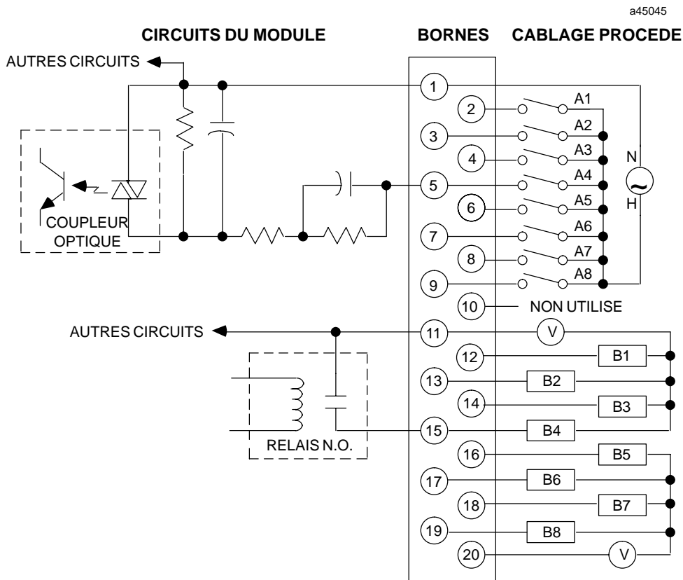
Figure 2-46. Câblage procédé - module d'entrée 120 Vca/sortie à relais - IC693MAR590
