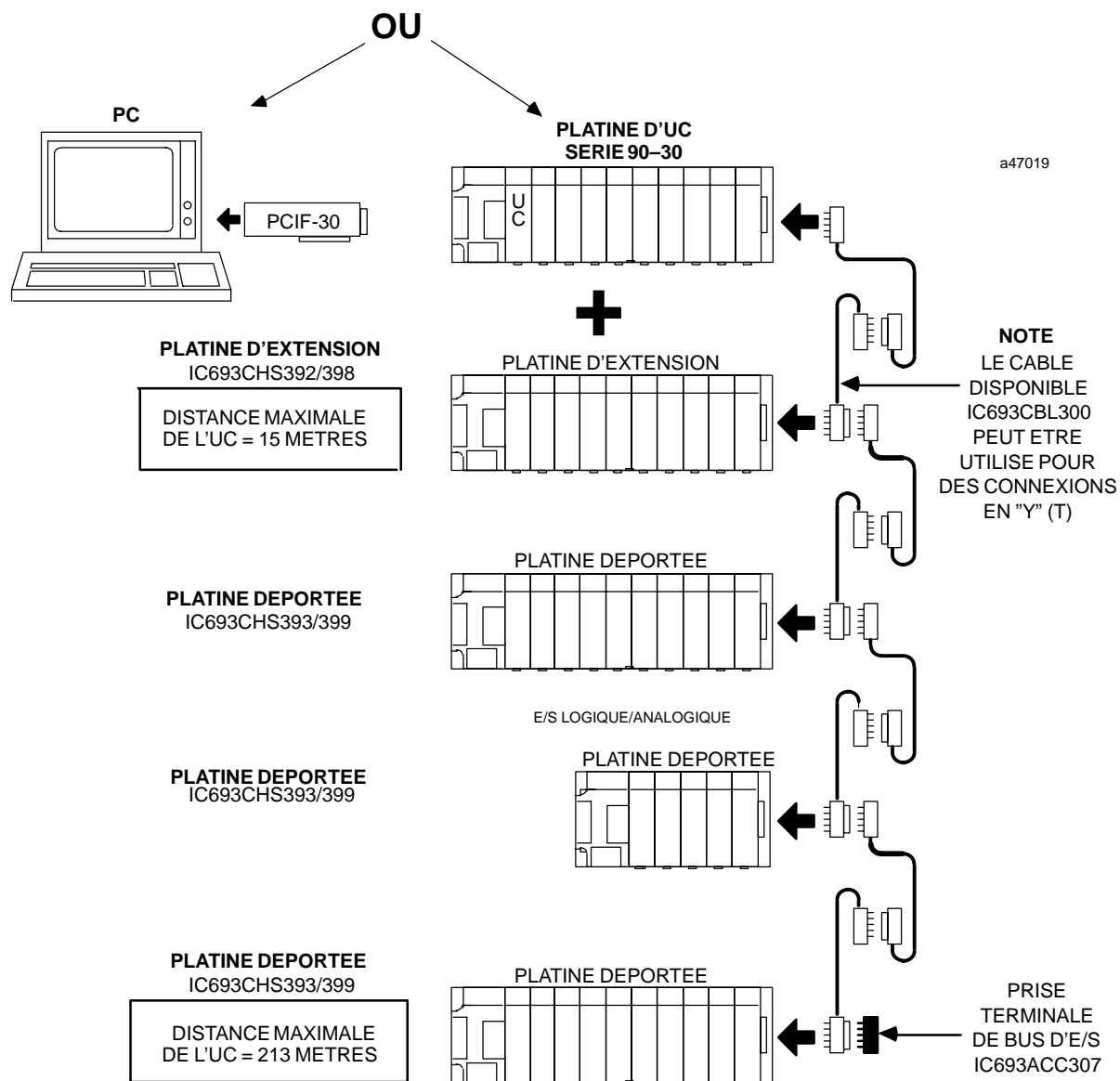
Figure 1-10. Exemple de connexion des platines dans un système d'extension d'E/S
