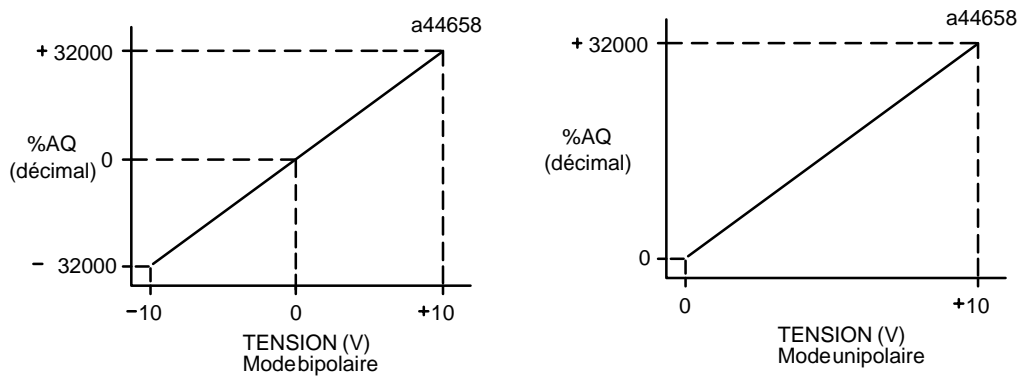
Figure 3-43. Mise à l'échelle de la sortie tension
