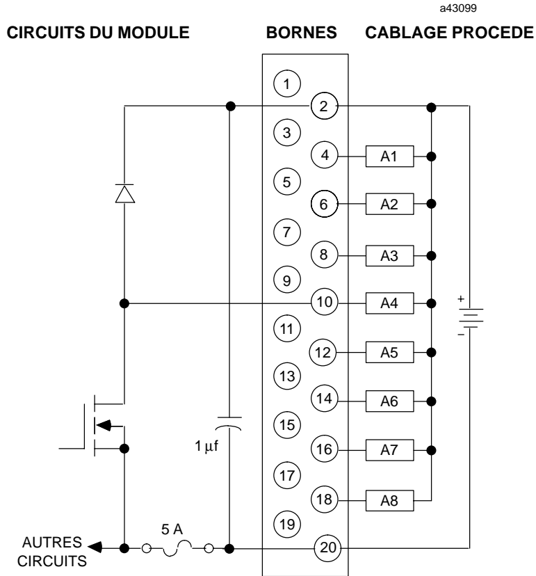
Figure 2-26. Câblage procédé - module de sortie logique négative 12/24 Vcc - 2 A - IC693MDL731
