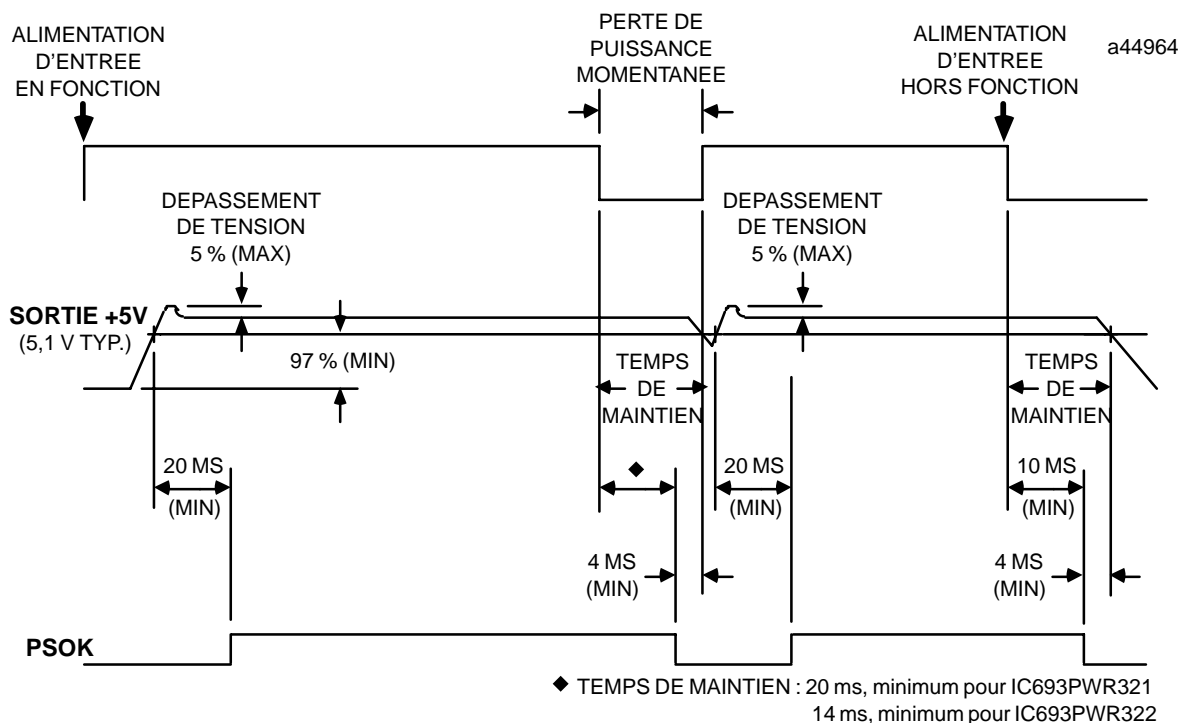
Figure 1-23. Chronogramme des alimentations Série 90-30
