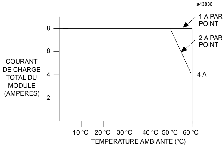
Figure 2-27. Courant de charge du module IC693MDL731 suivant la température
