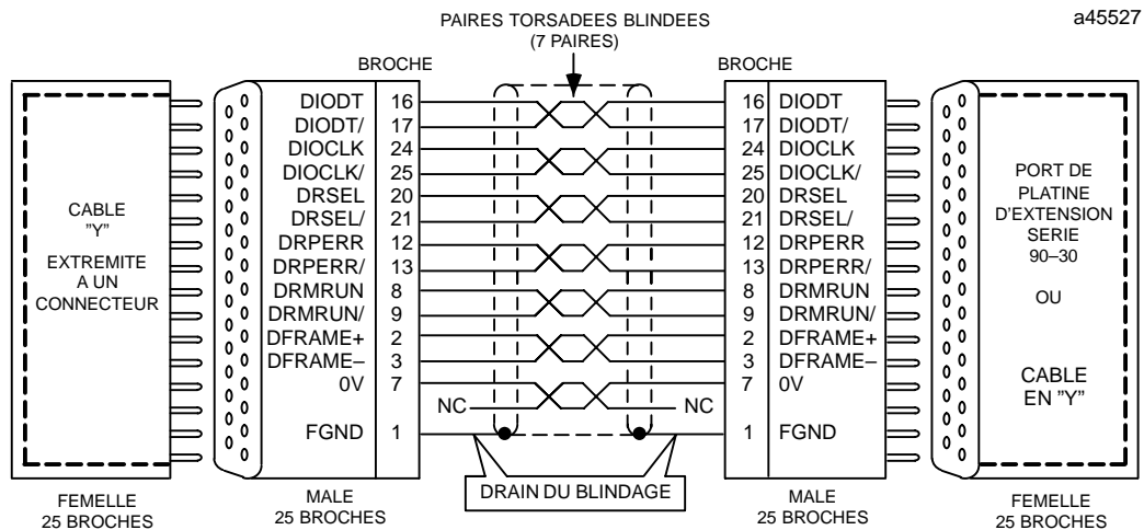
Figure C-2. Schéma de câblage point-à-point pour les applications nécessitant une insensibilité au bruit moins importante
