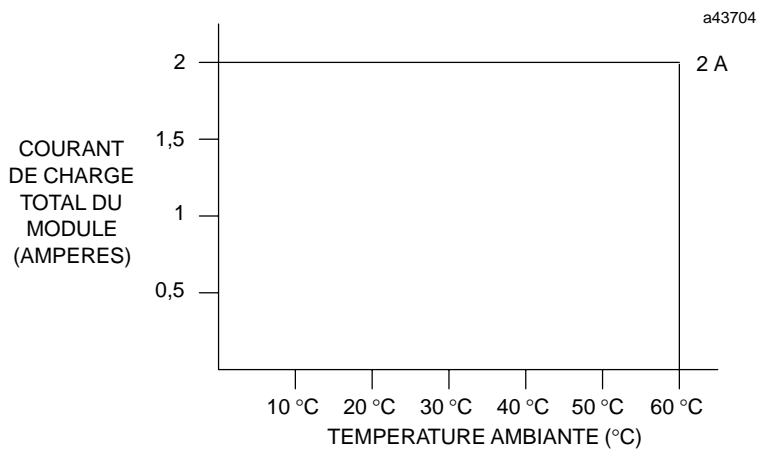
Figure 2-29. Courant de charge du module IC693MDL732 suivant la température
