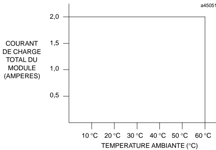
Figure 2-31. Courant de charge en fonction de la température pour le module IC693MDL733
