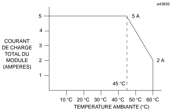
Figure 2-23. Courant de charge du module IC693MDL390 suivant la température
