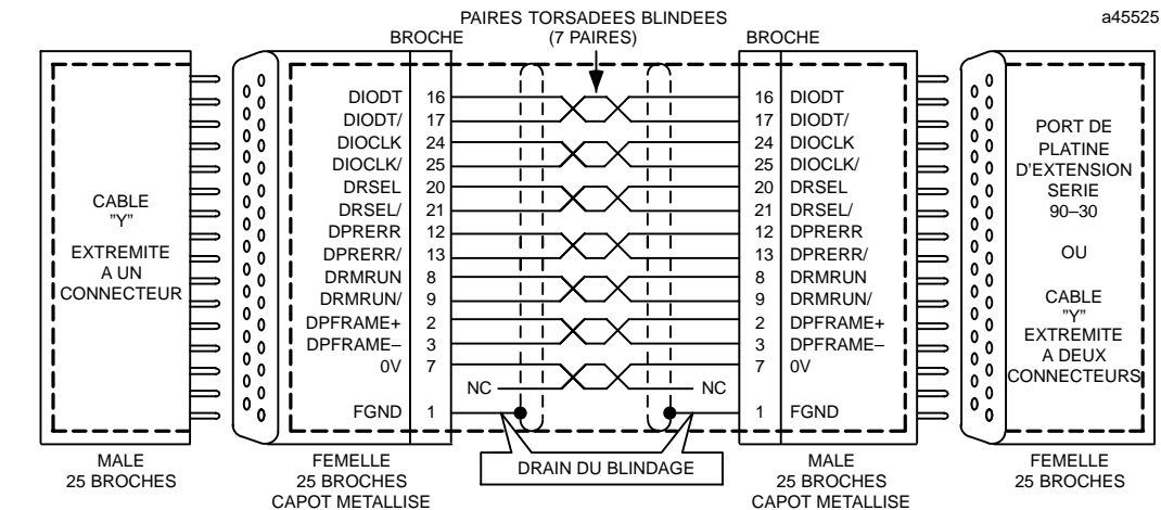
Figure 1-12. Platine d'extension (CHS392/398) Schéma de câblage point-à-point
