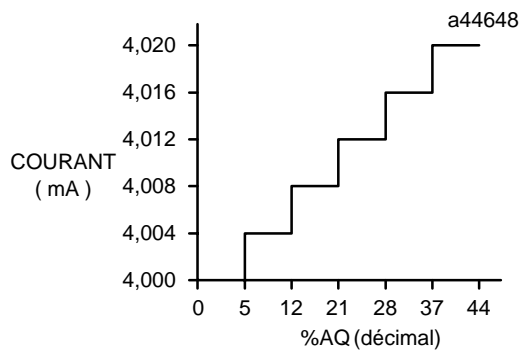
Figure 3-5. Effet marche d'escalier sur les valeurs analogiques
