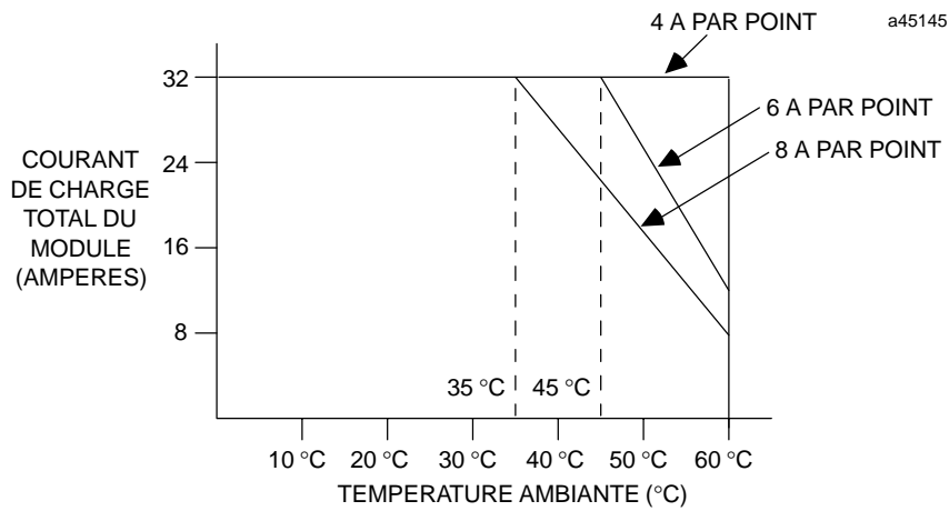
Figure 2-43. Courant de charge du module IC693MDL931 suivant la température
