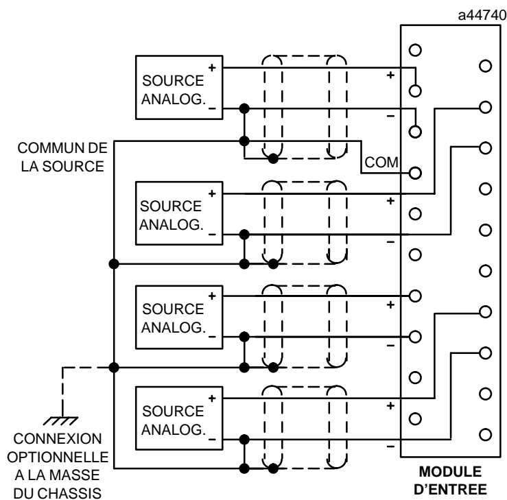
Figure 3-8. Connexion du blindage pour les modules d'entrée analogiques
