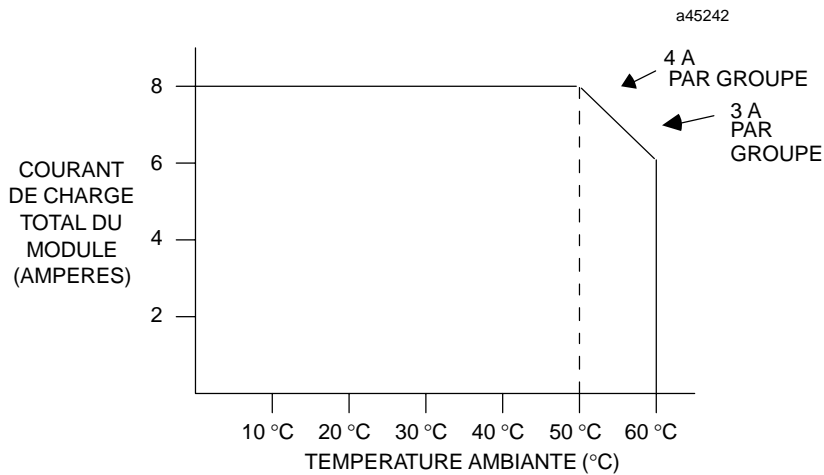
Figure 2-39. Courant de charge du module IC693MDL742 suivant la température
