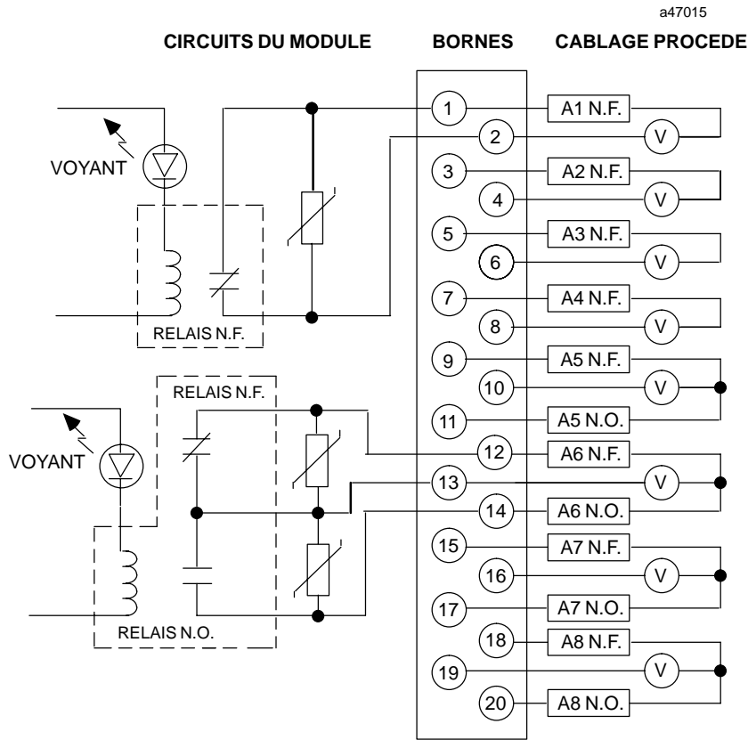
Figure 2-42. Câblage procédé - module de sortie à relais isolée, N.F. et en forme de C - 8 A - IC693MDL931
