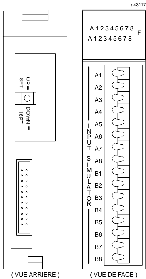
Figure 2-15. Module simulateur d'entrées
