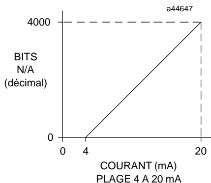
Figure 3-34. Bits N/A en fonction de la sortie de courant, 4 à 20 mA
