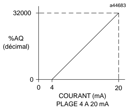
Figure 3-36. Mise à l'échelle de la sortie de courant, 4 à 20 mA
