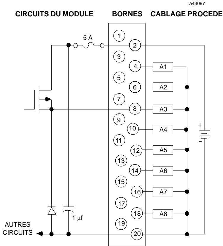
Figure 2-24. Câblage procédé - module de sortie logique positive 12/24 Vcc - 2 A - IC693MDL730
