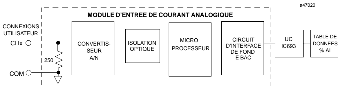
Figure 3-25. Schéma fonctionnel du module d'entrée de courant analogique 16 voies - IC693ALG223
