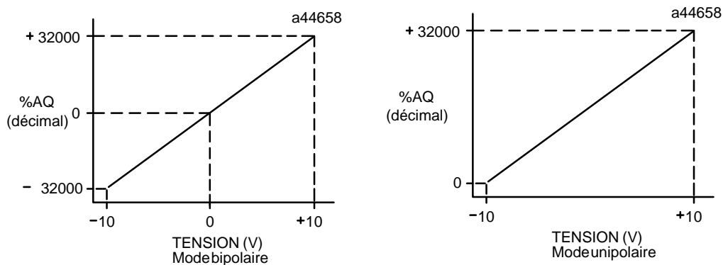
Figure 3-51. Mise à l'échelle de la sortie tension
