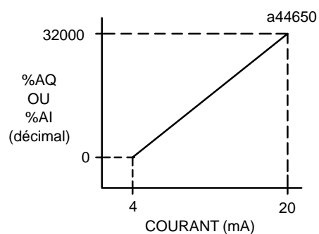
Figure 3-7. Courant en fonction du mot de donnée
