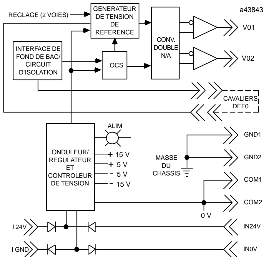
Figure 3-32. Schéma fonctionnel du module de sortie de tension analogique - IC693ALG390
