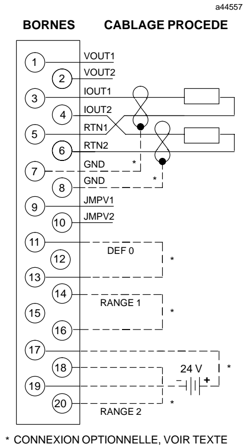
Figure 3-40. Câblage procédé - module de sortie de courant analogique (mode courant) - IC693ALG391
