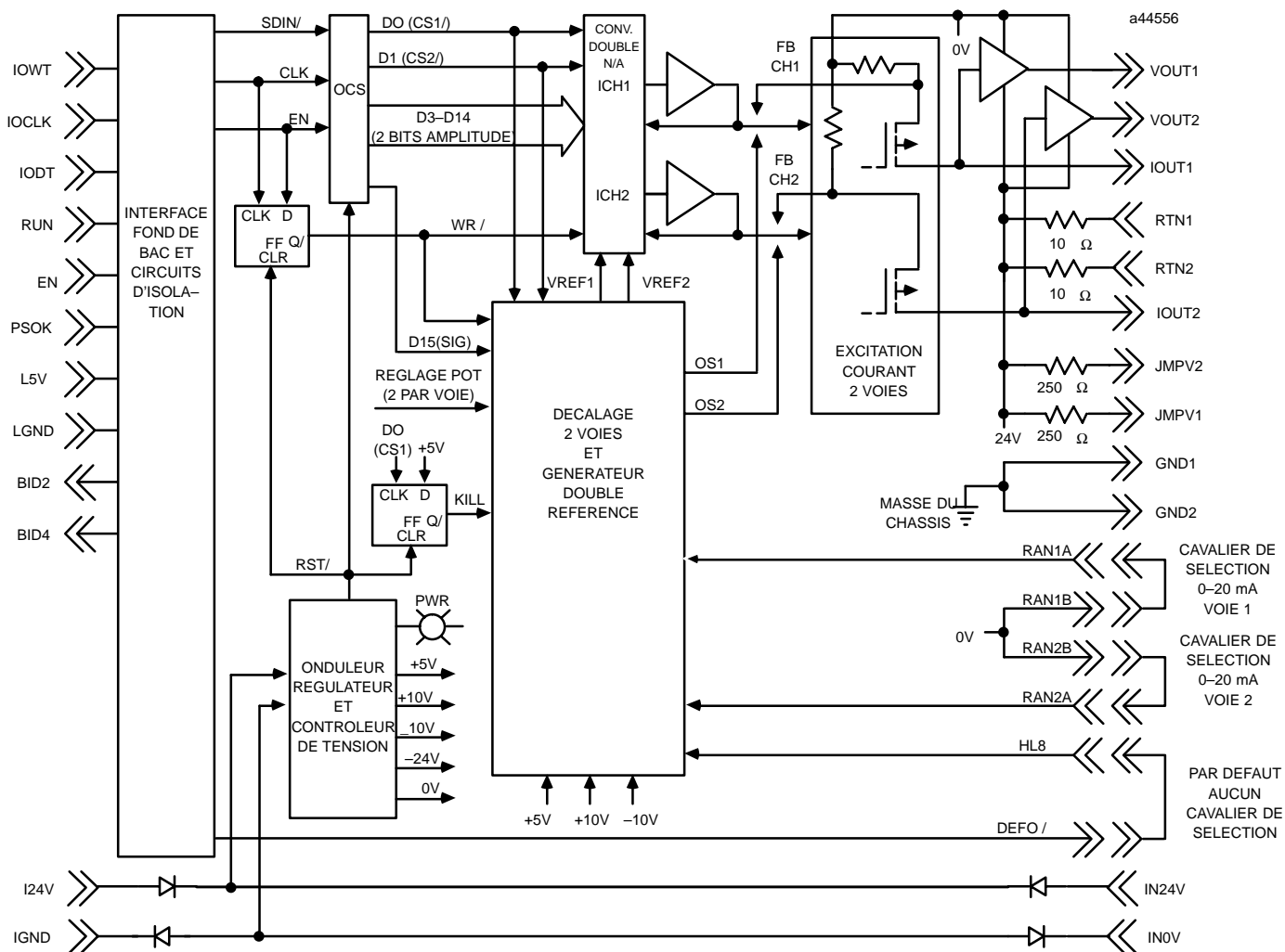
Figure 3-39. Schéma fonctionnel du module de sortie de courant analogique - IC693ALG391
